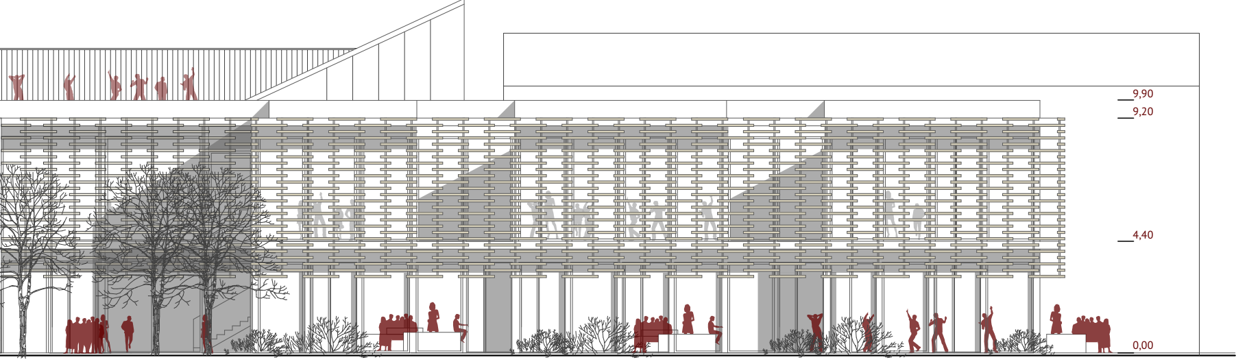
ZAHODNA FASADA OSNOVNE ŠOLE merilo 1:200
