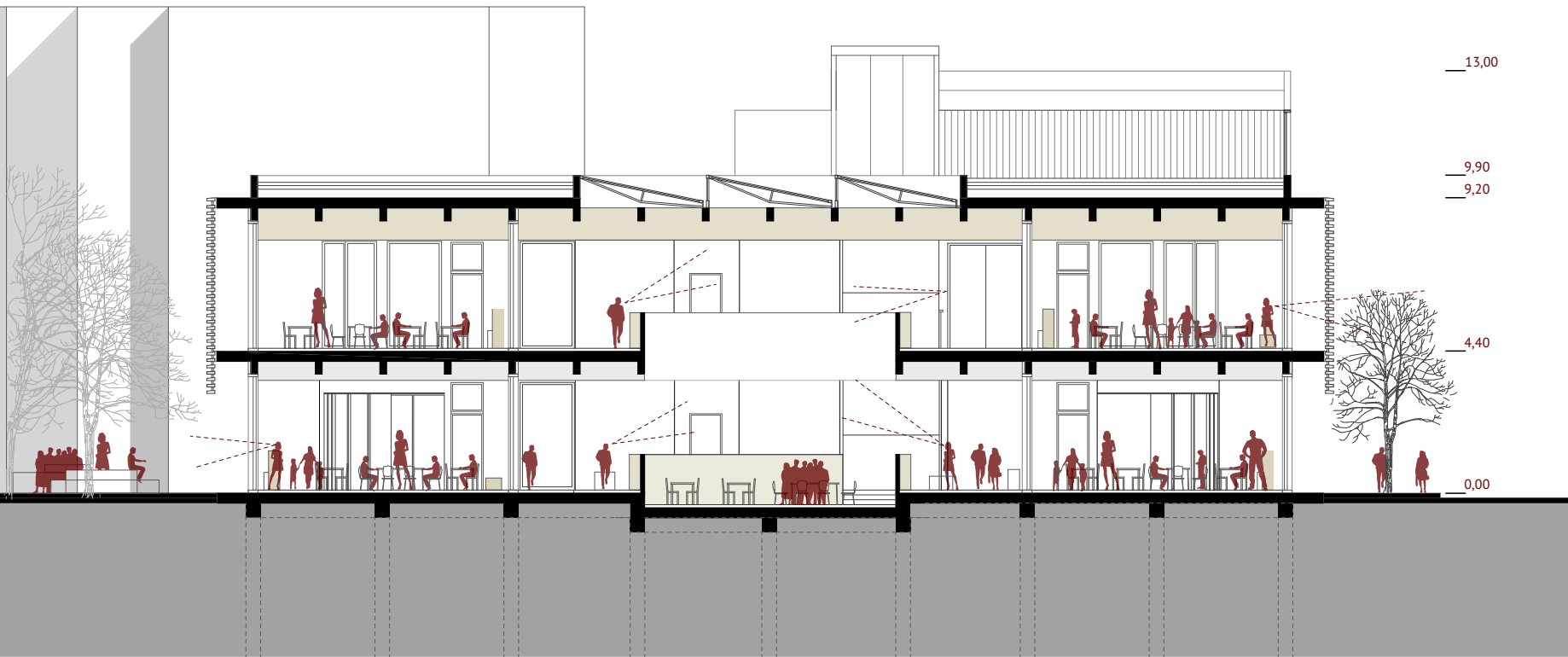
PREREZ A-A OSNOVNE ŠOLE merilo 1:200
