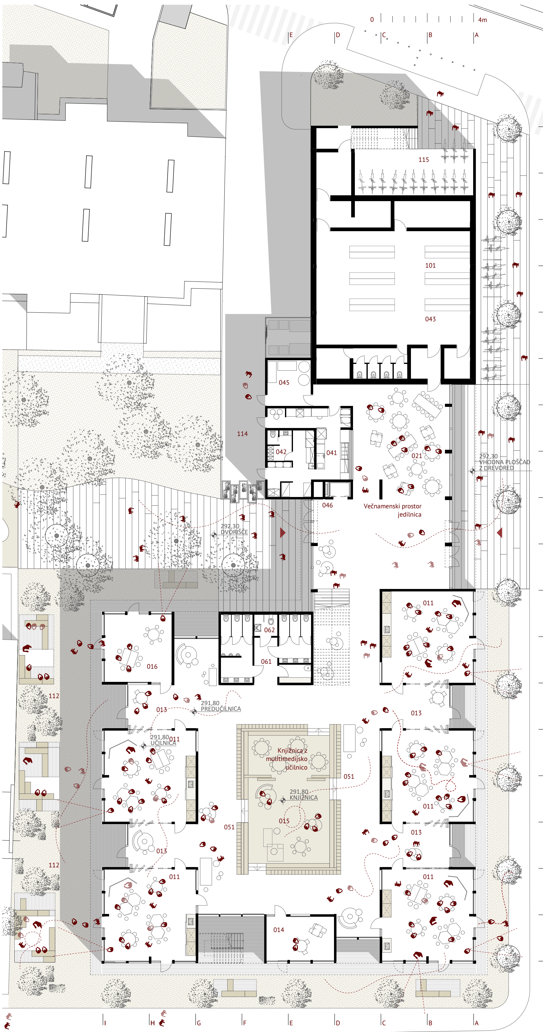
TLORIS PRITLIČJA OSNOVNE SOLE merilo 1:200
