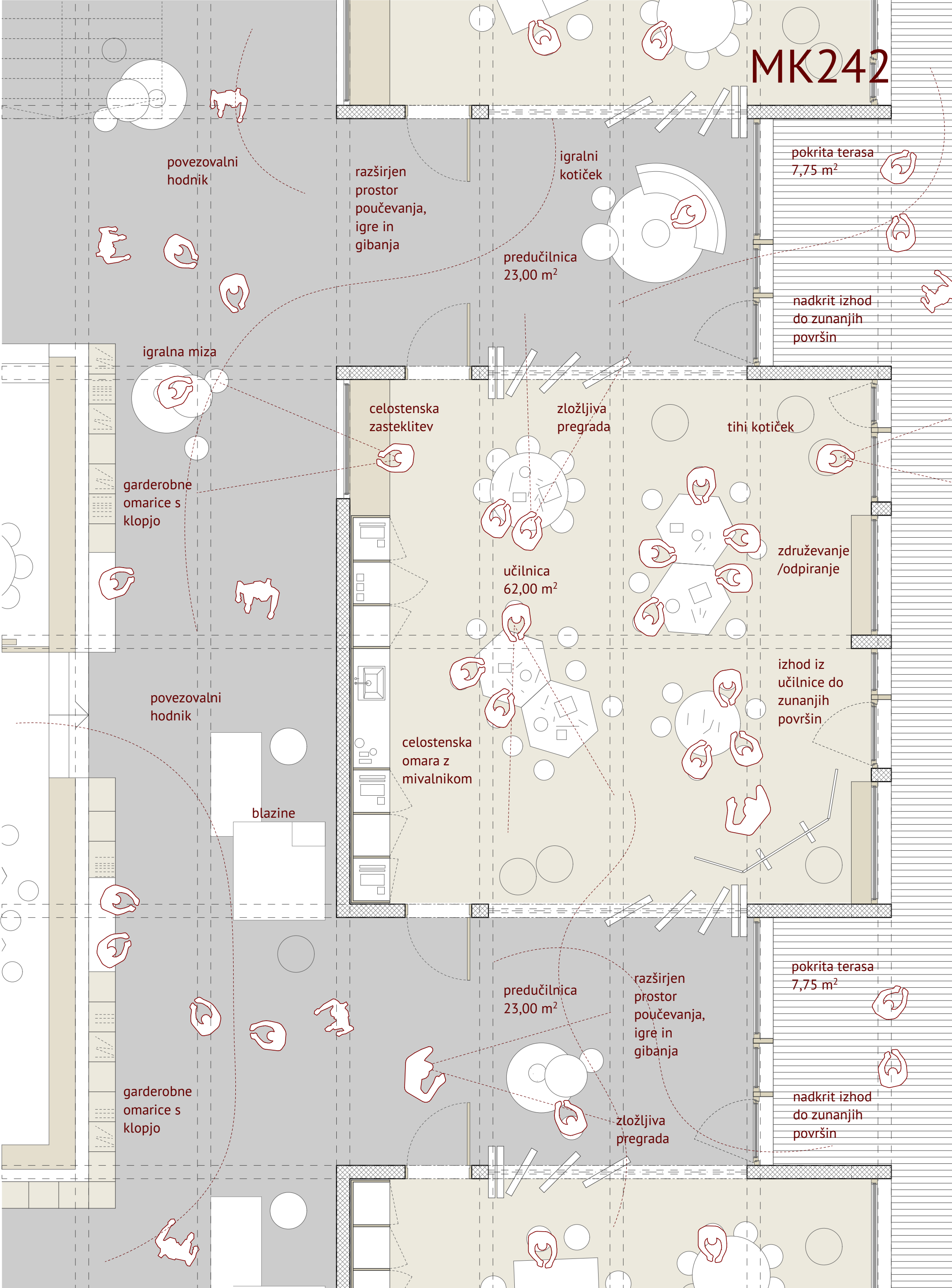
TLORIS UČILNICE S PREDUČILNICO merilo 1:50
