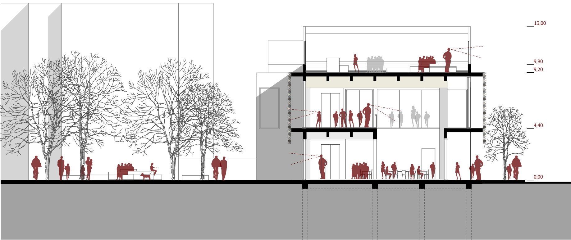
PREREZ B-B OSNOVNE ŠOLE merilo 1:200
