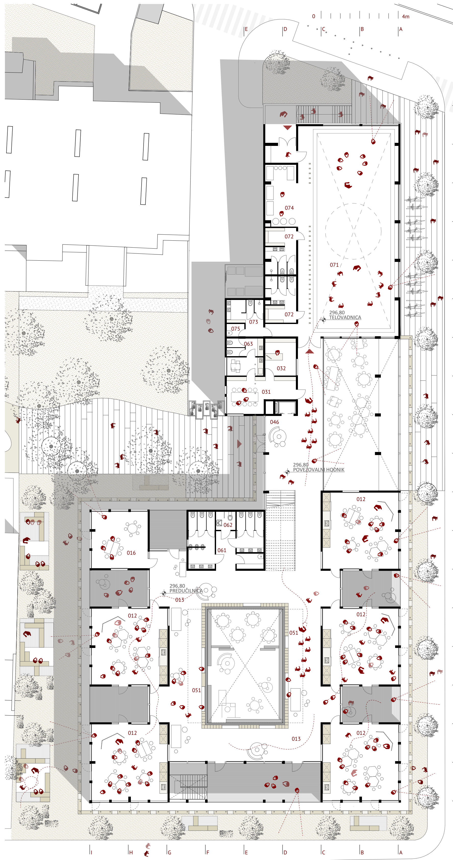
TLORIS PRITLIČJA OSNOVNE SOLE merilo 1:200
