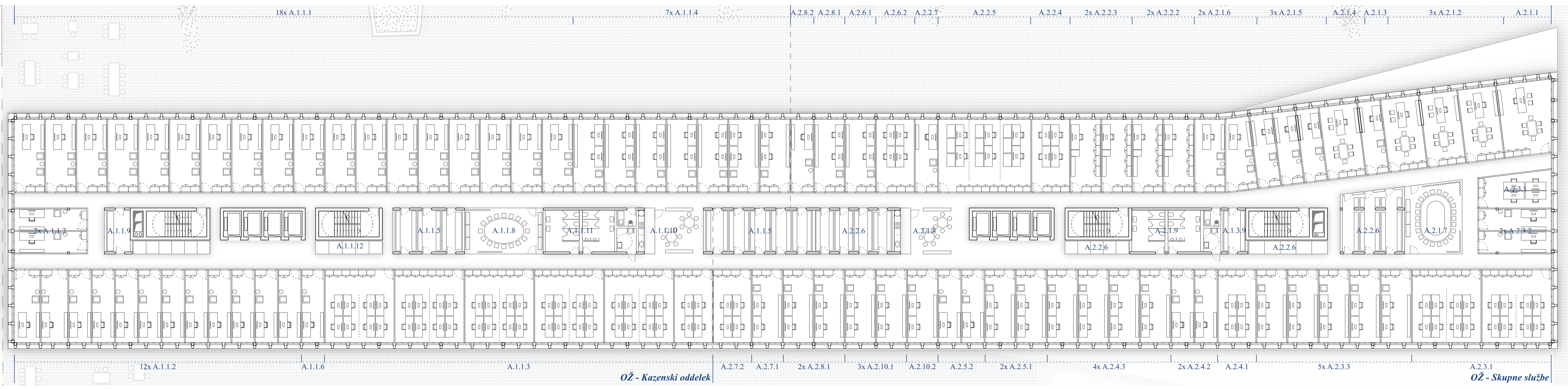
tloris 6. etaže m 1:250
