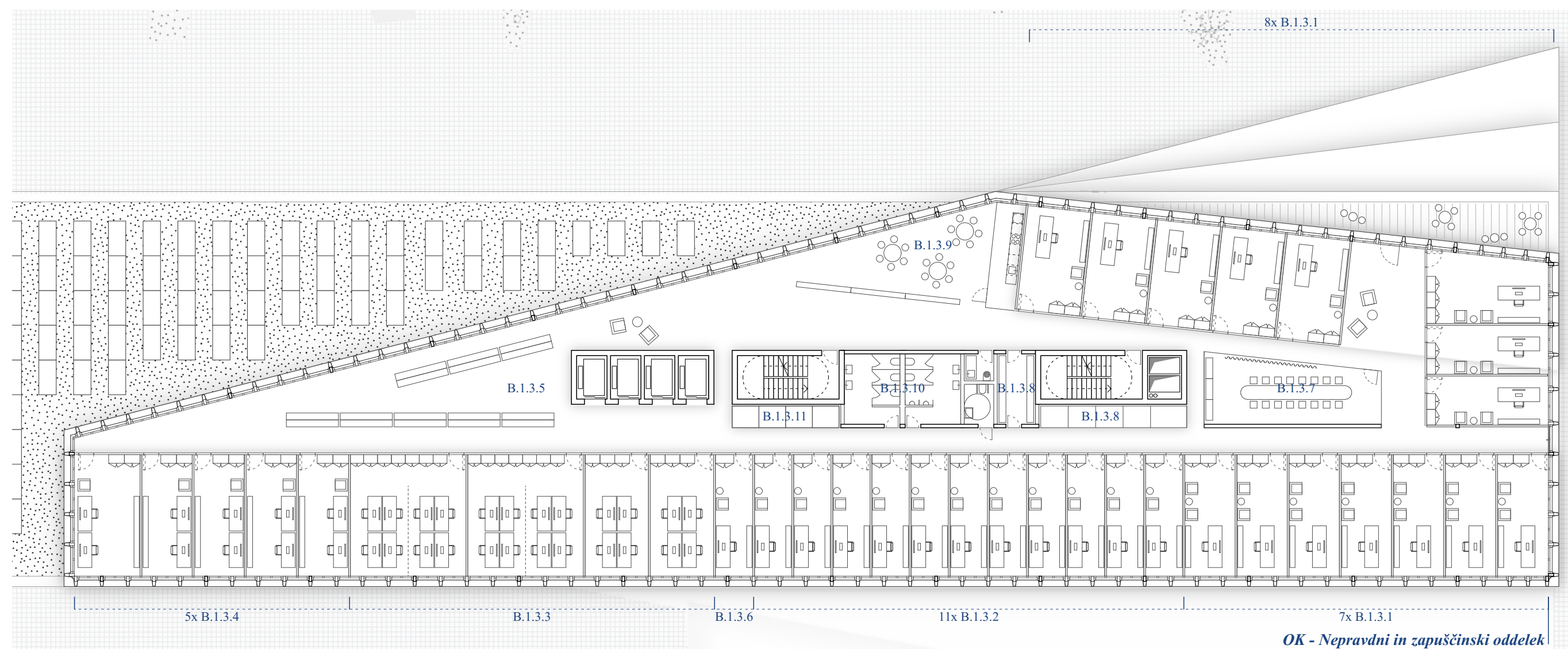
tloris 10. etaže m 1:250
