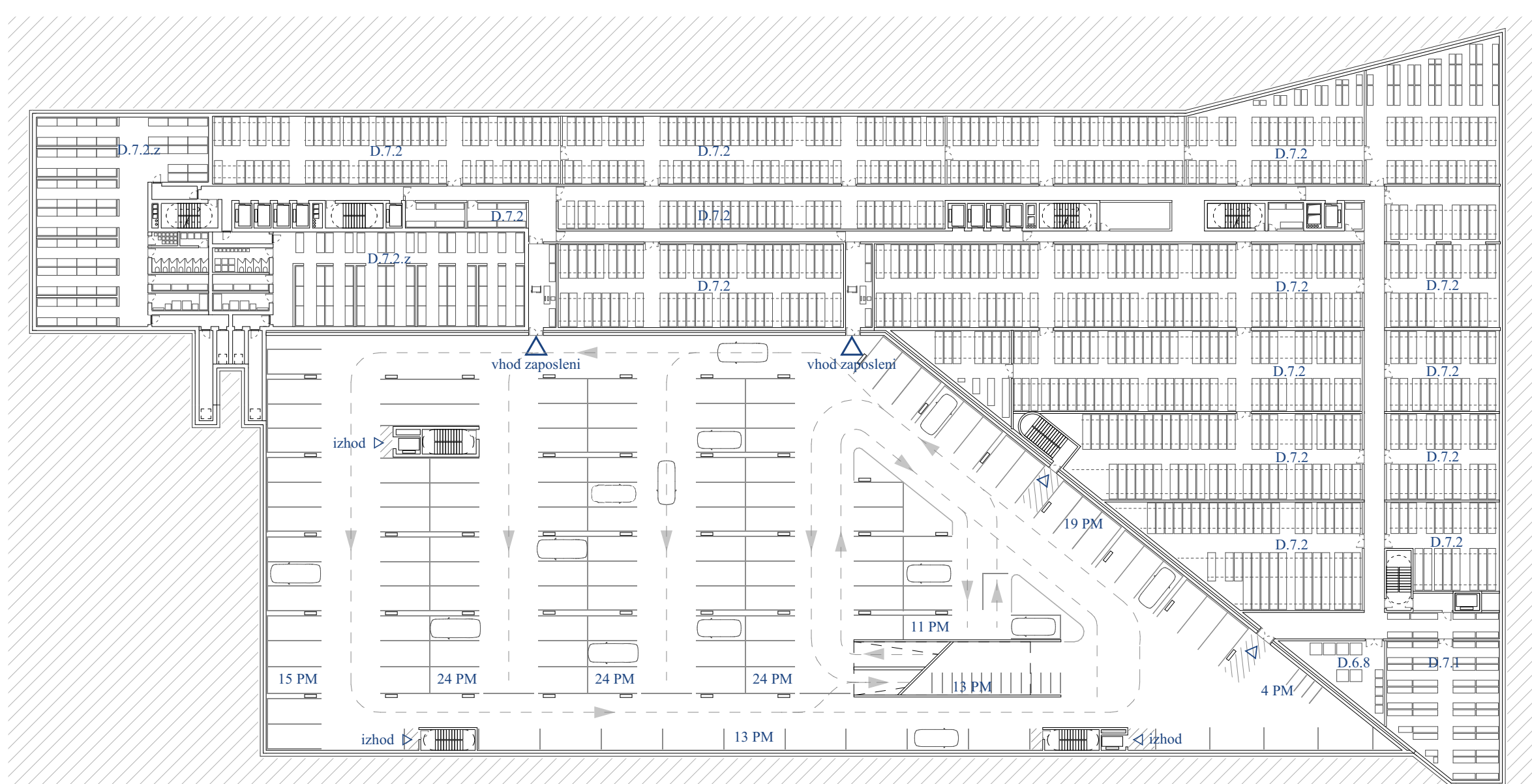
tloris 3. kletne etaže m 1:250
