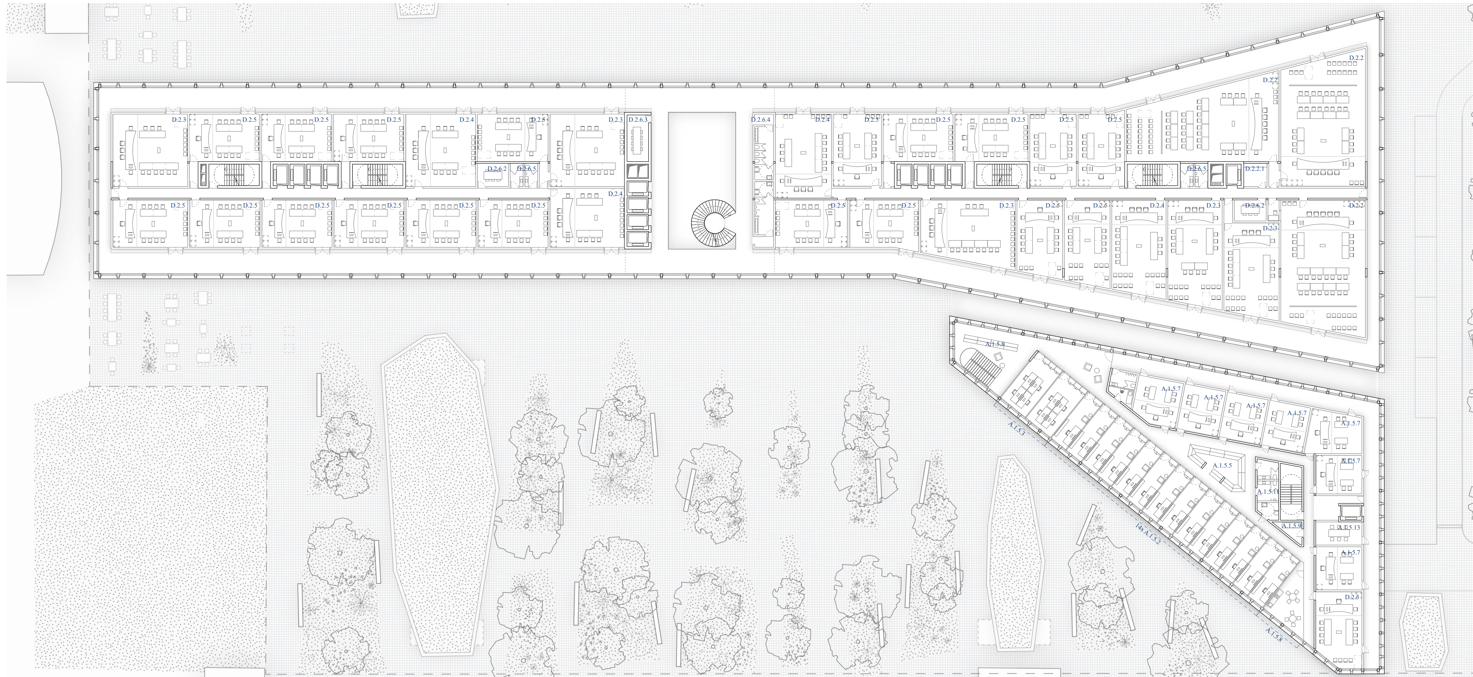
tloris 1. etaže
