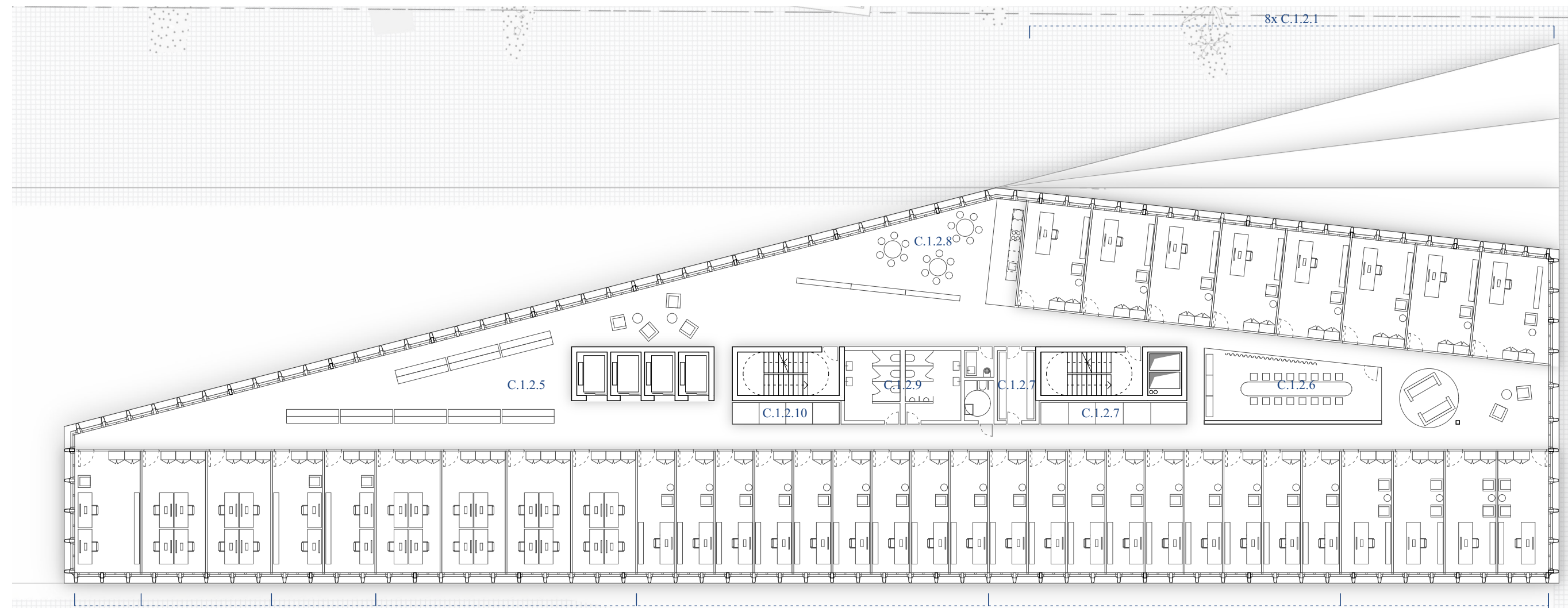
tloris 12. etaže m 1:250
