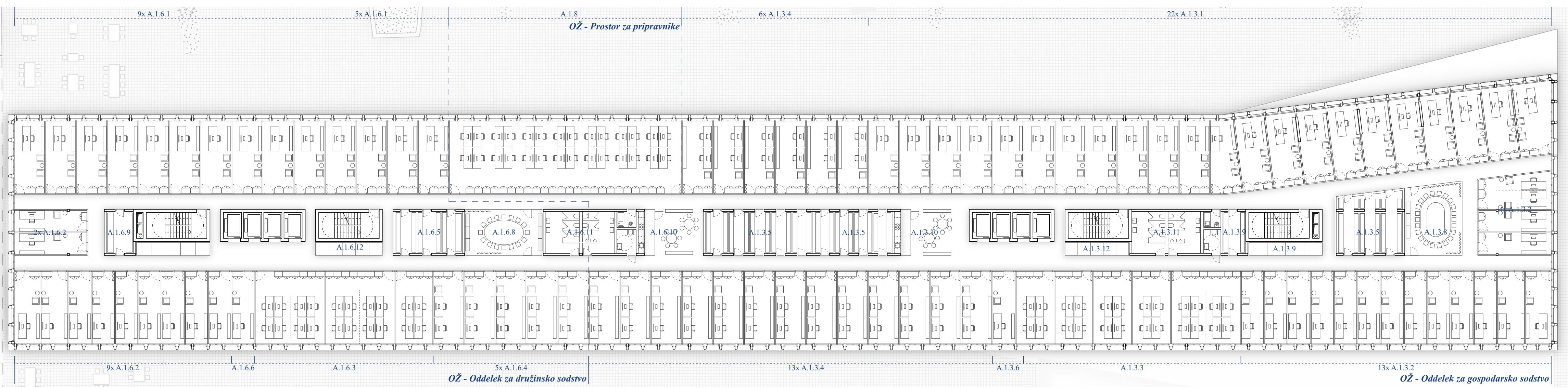
tloris 5. etaže m 1:250
