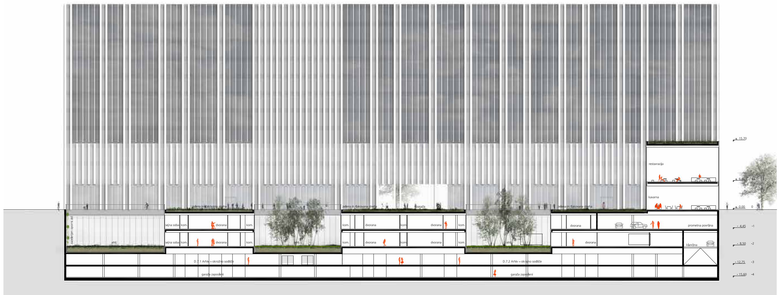
ZAHODNA FASADA
