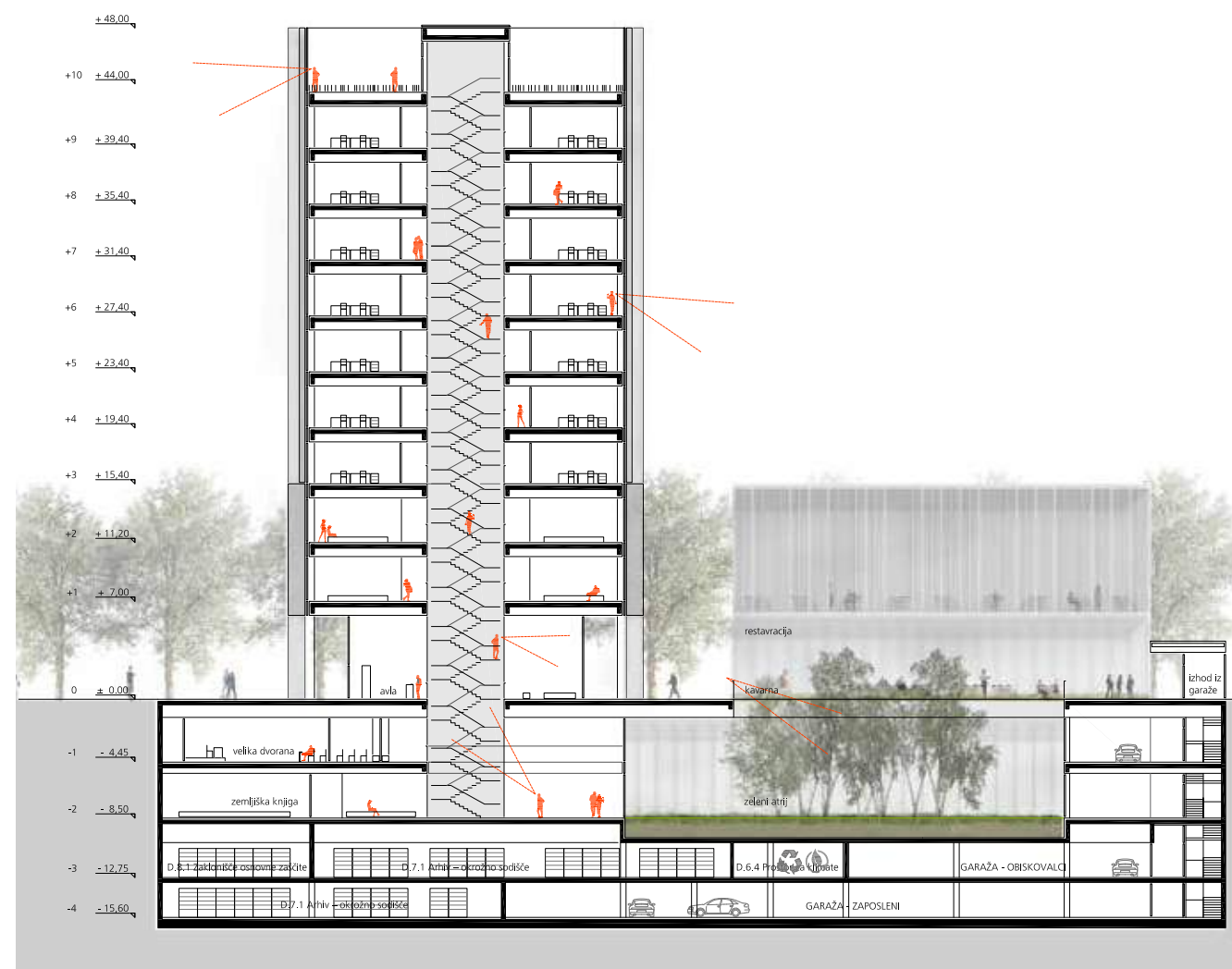
PREREZ B-B
