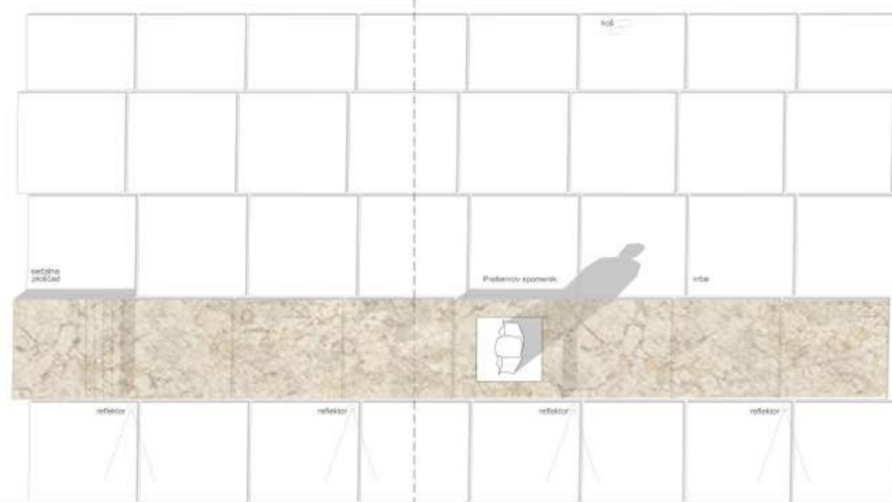
SEGMENT TLAKOVANJA PRED PREŠERNOVIM GLEDALIŠČEM KRANJ tloris_1:100
