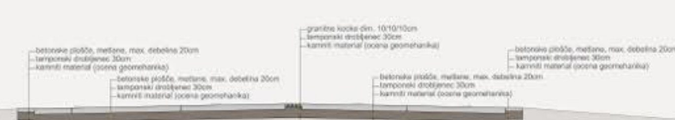
SEGMENT TLAKOVANJA GLAVNI TRG, POŠTNA ULICA pano 03
