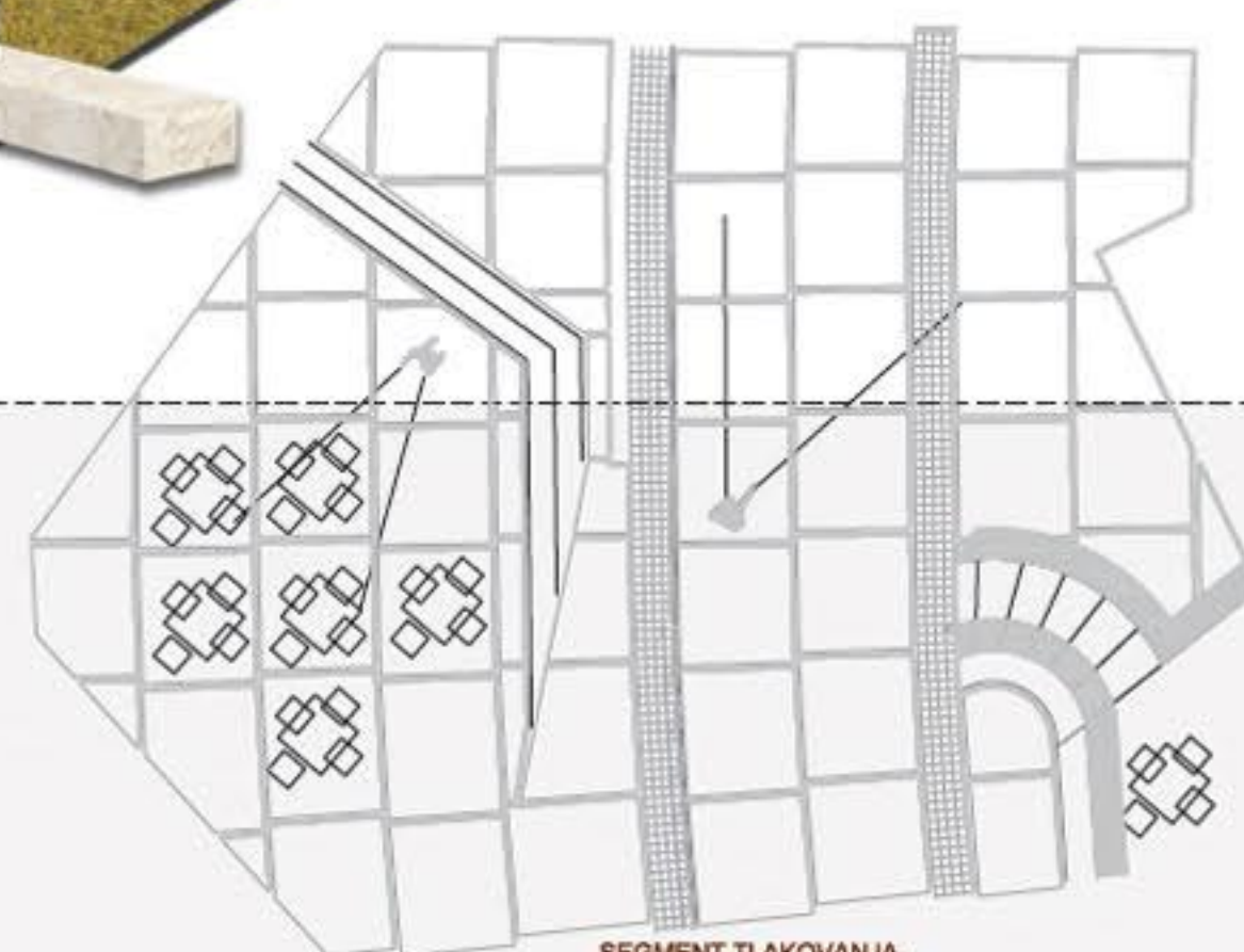
SEGMENT TLAKOVANJA NA VODOPIVČEVI ULICI tloris in prerez_1:100
