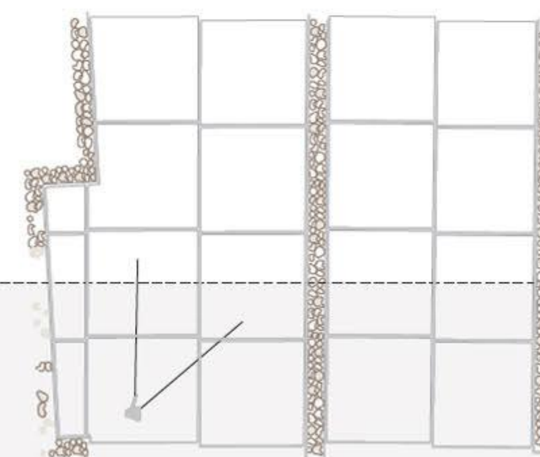
SEGMENT TLAKOVANJA TRUBARJEV TRG tloris in prerez_1:100
