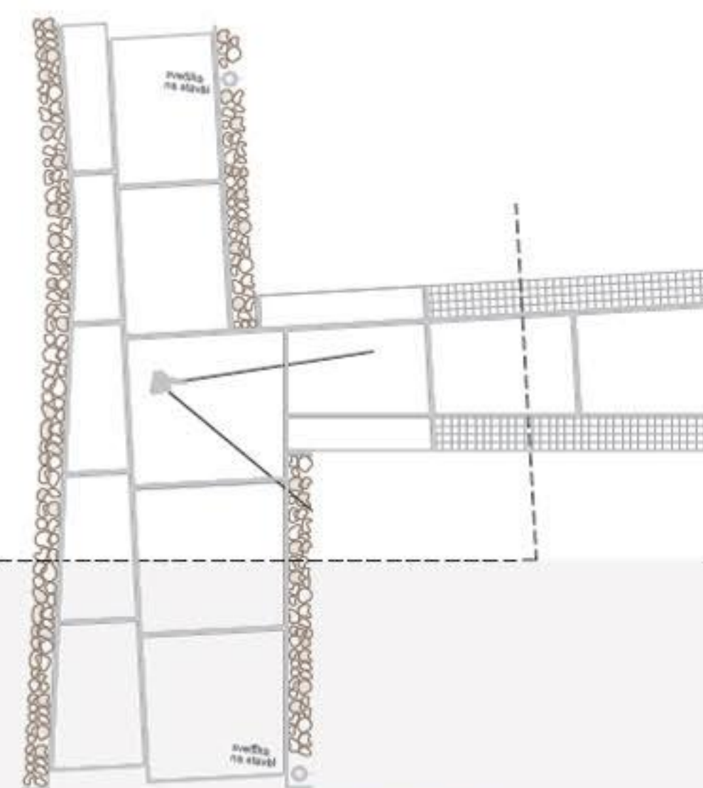
SEGMENT TLAKOVANJA NA STIKU CANKARJEVE IN TOMŠIČEVE ULICE tloris in prerez_1:100
