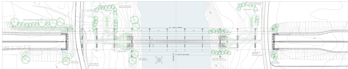
TLORIS MOSTU 5-03 M 1:500
