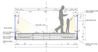
KARAKTERISTIČNI PREČNI PREREZ MOSTU 5-03 M 1:25
