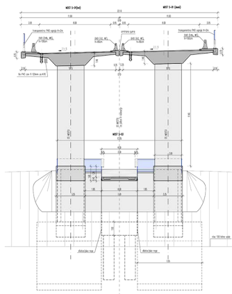
PREČNI PREREZ MOSTOV 5-01 in 5-03 M 1:100
