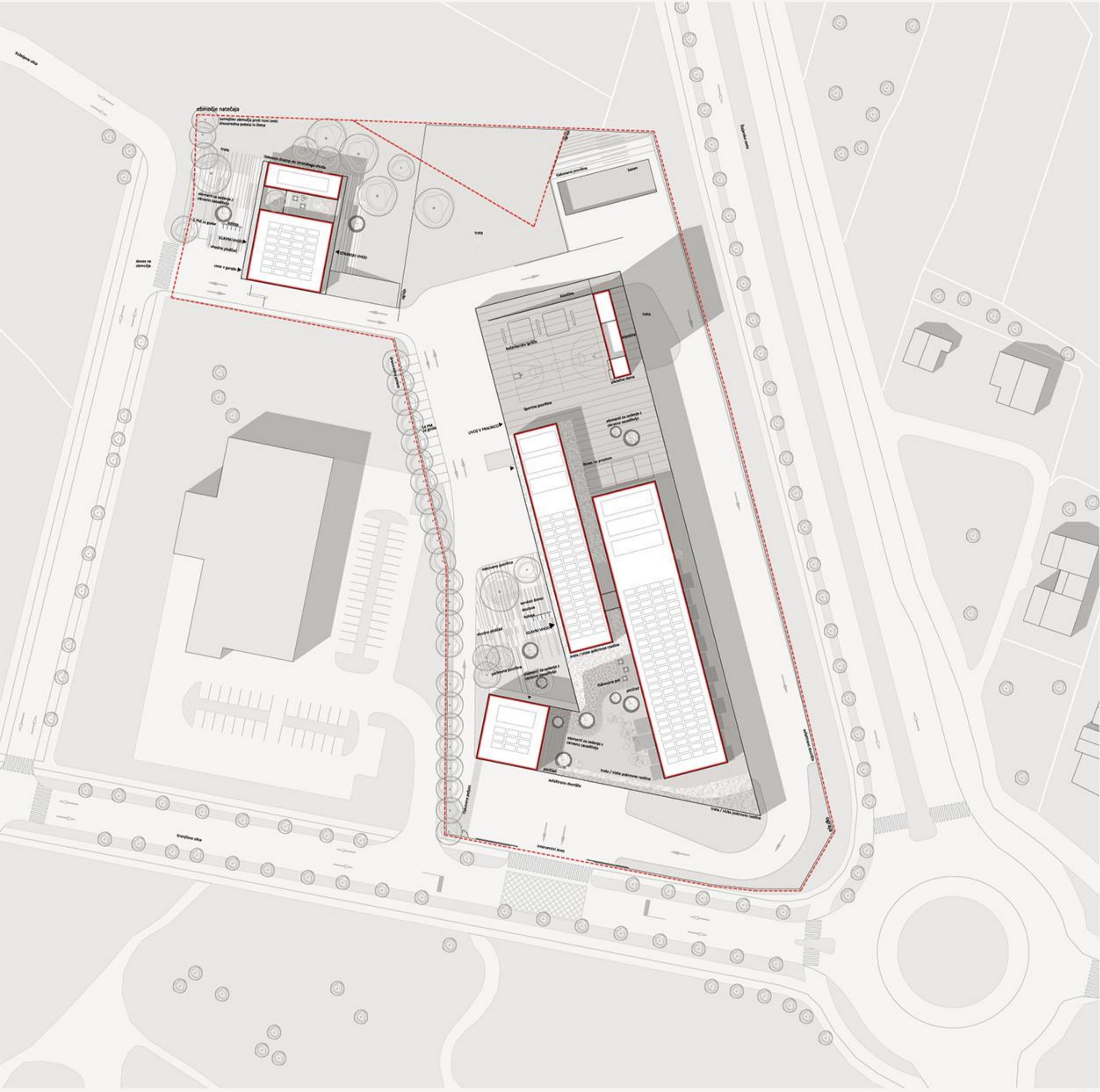
SITUACIJA UREDITVE OBMOČJA M 1:500
