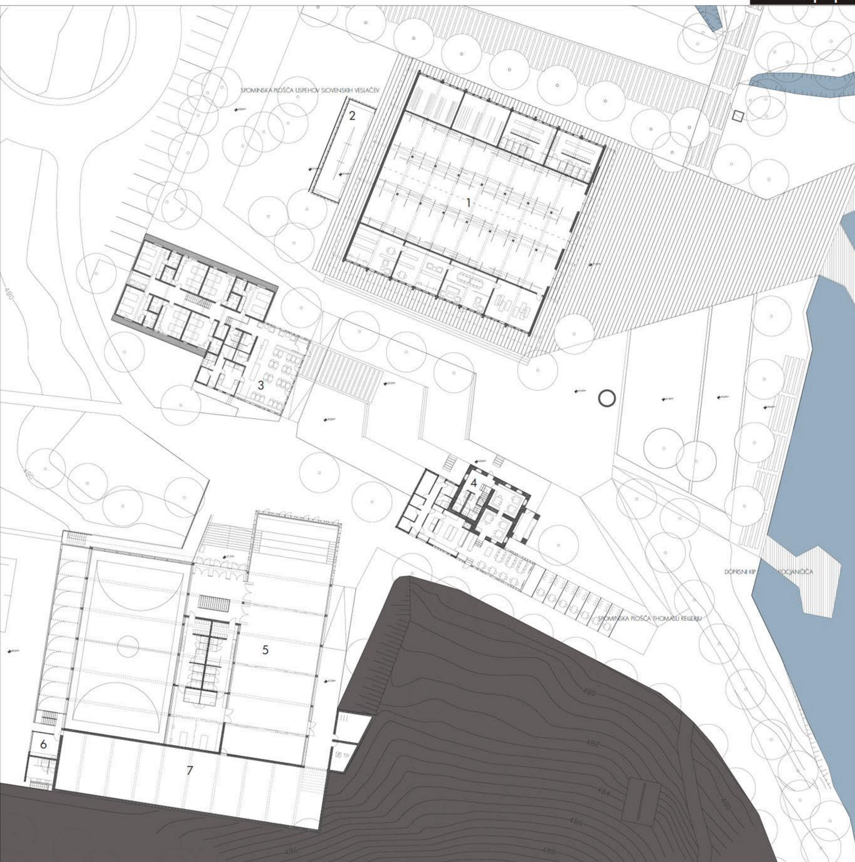
SITUACIJA_TLORIS PRITLIČJA_M_1_200
