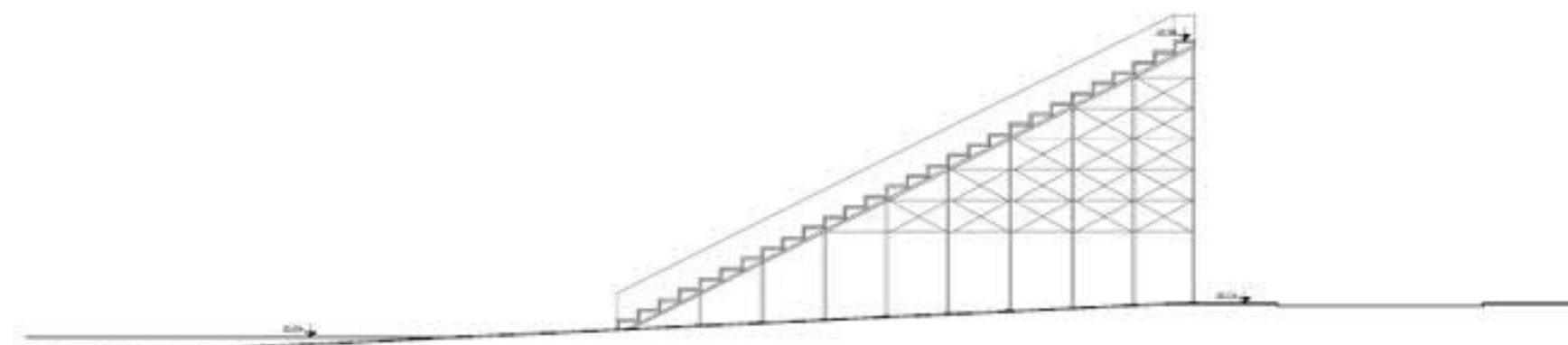
ZAČASNE TRIBUNE ZAHOD_SHEMATSKI PREREZ_M_1_200
