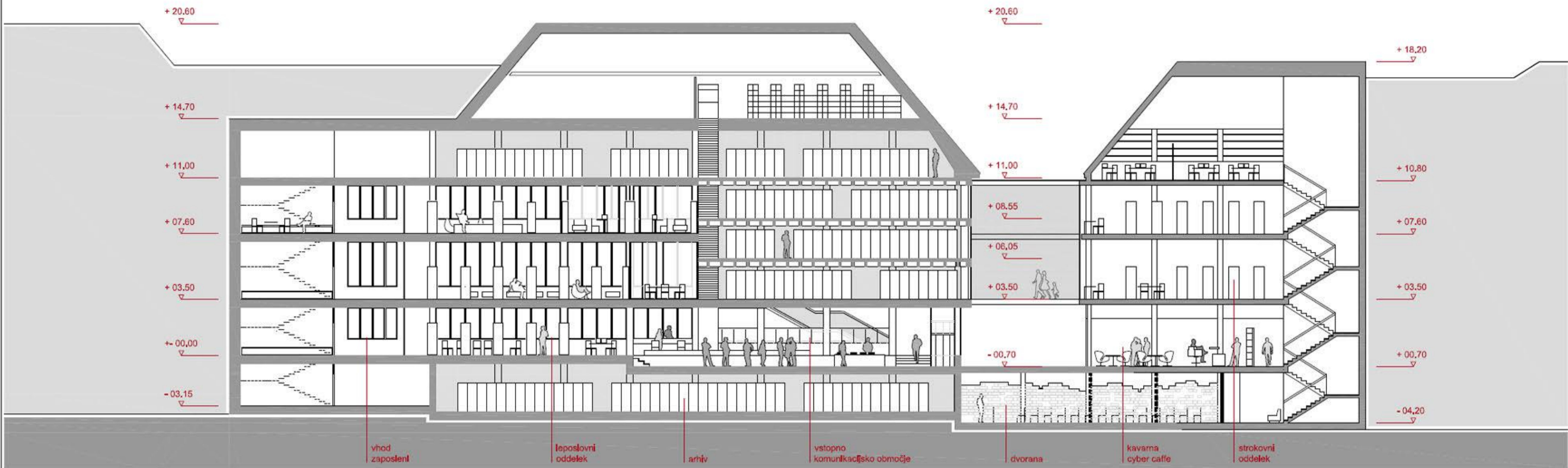
PREREZ BB 1:100
