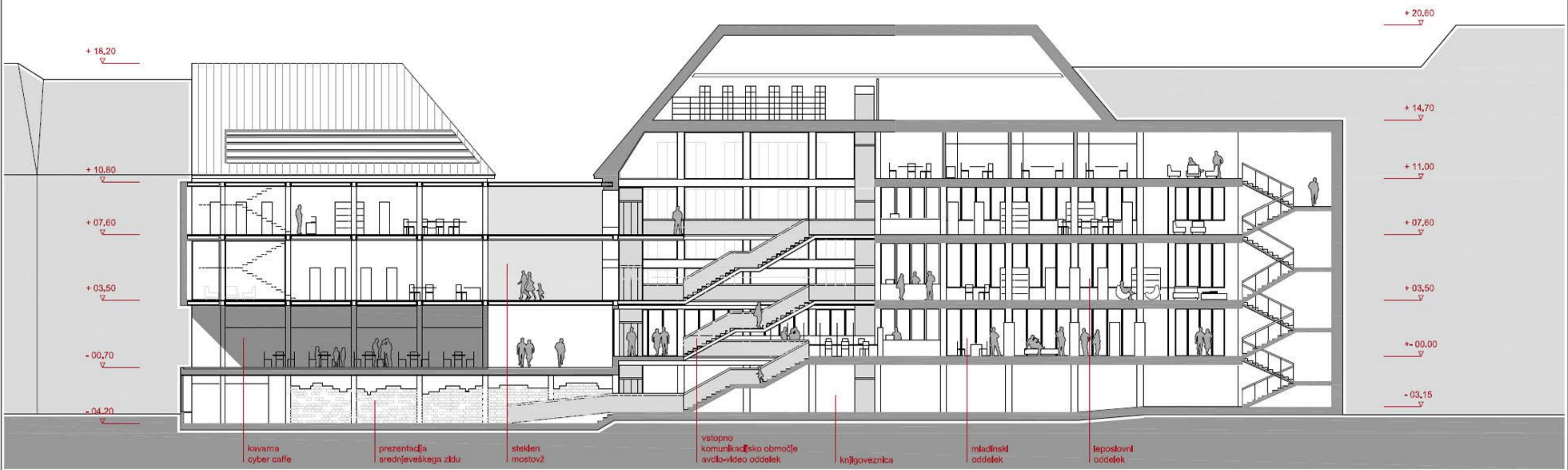
PREREZ AA 1:100
