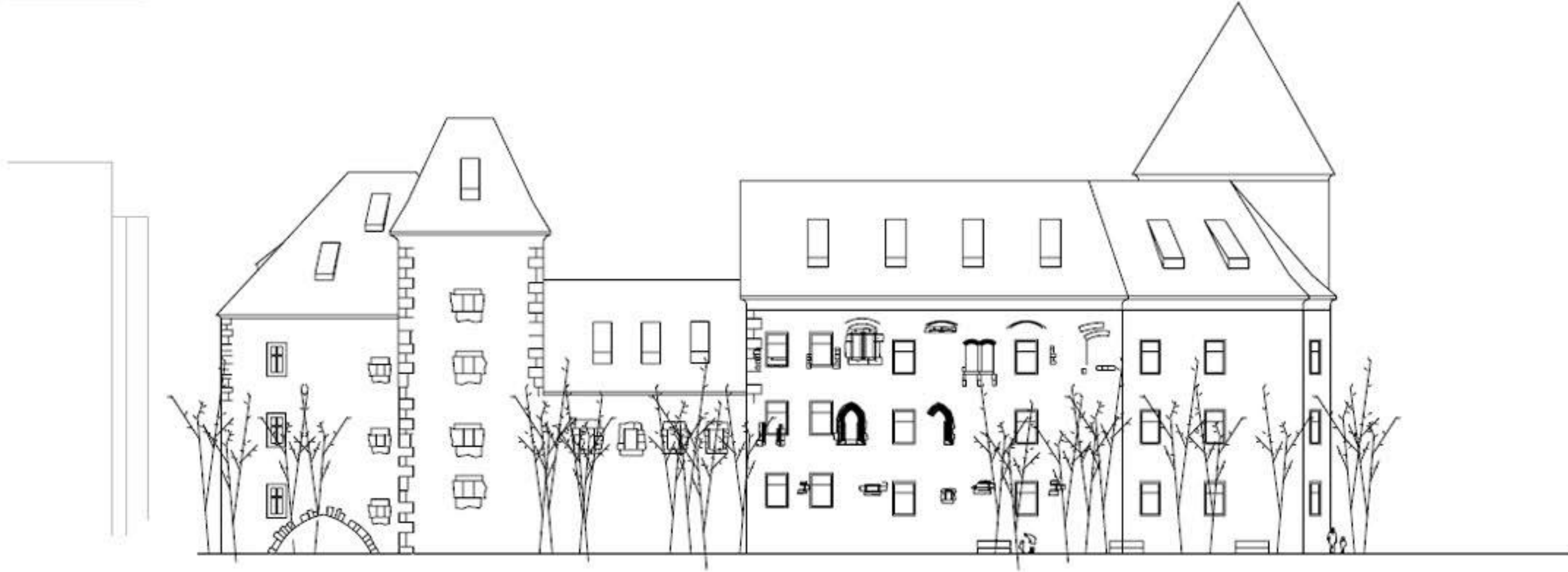
ZAHODNA FASADA, M1/200
