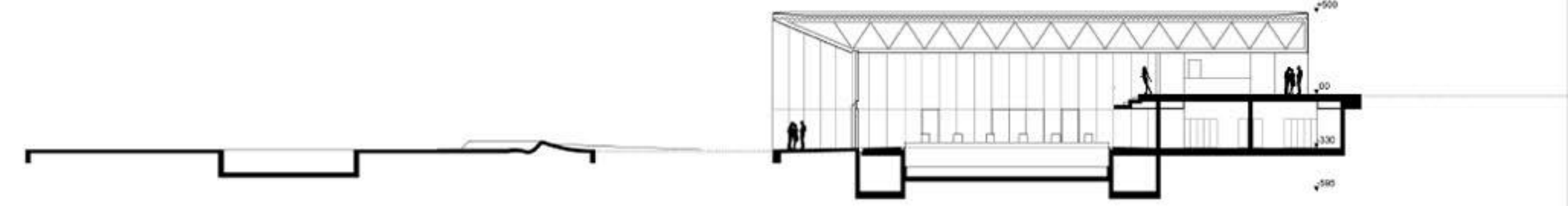
PREREZ 4-4
