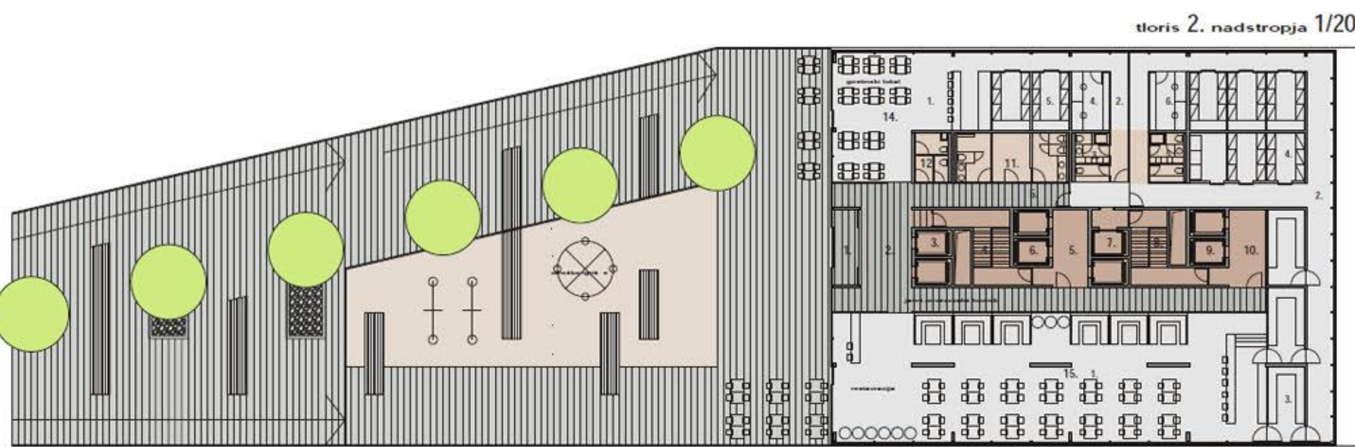
tloris 2. nadstropja 1/200
