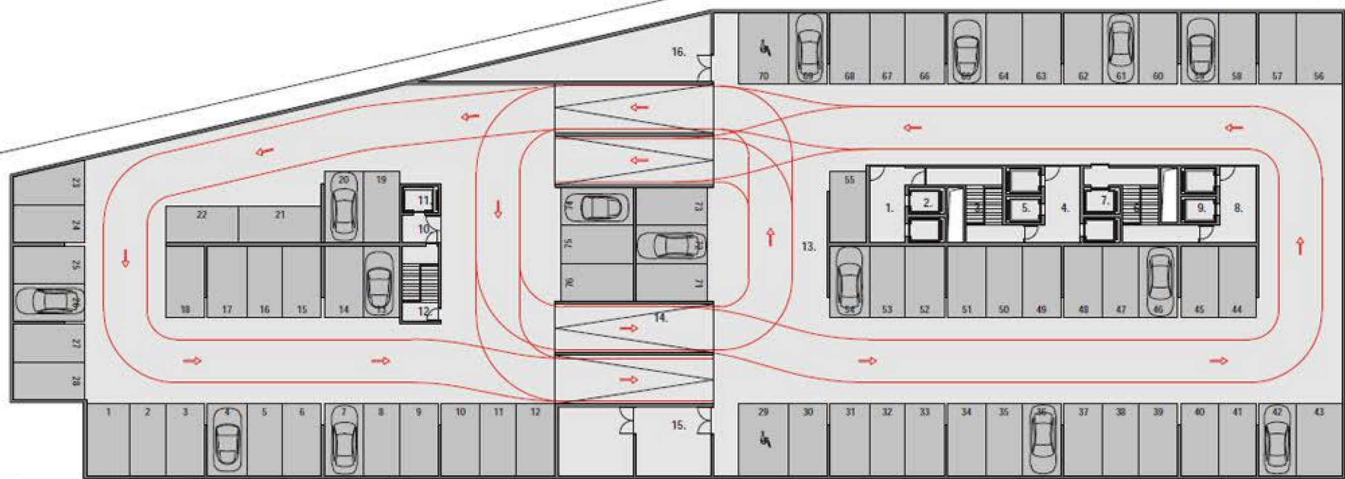
tloris 2.-6. kleti 1/200
