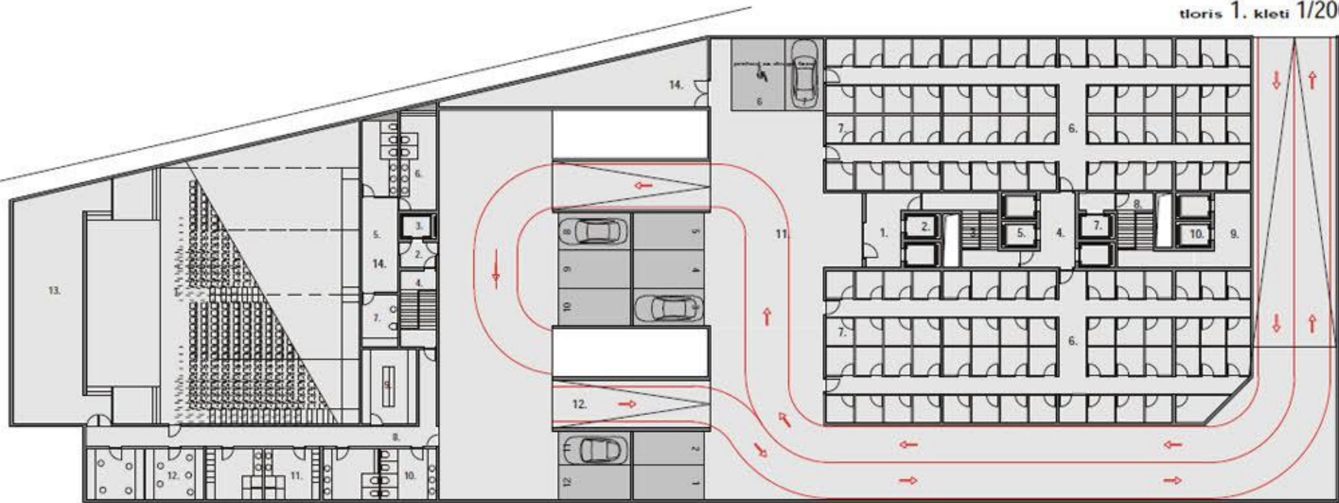
tloris 1. kleti 1/200
