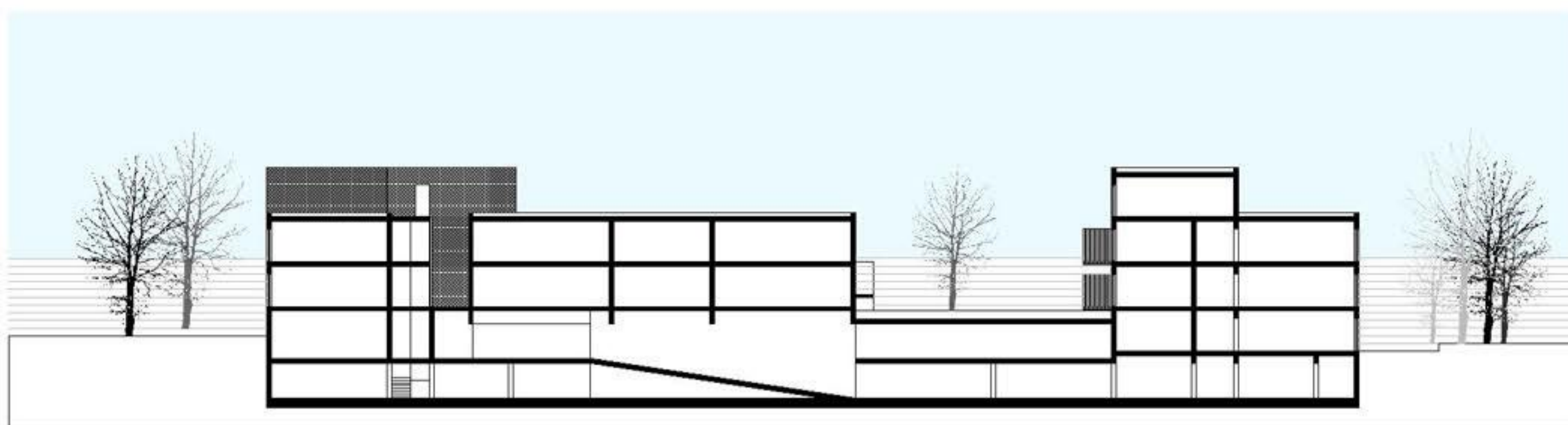
PREREZ BB
