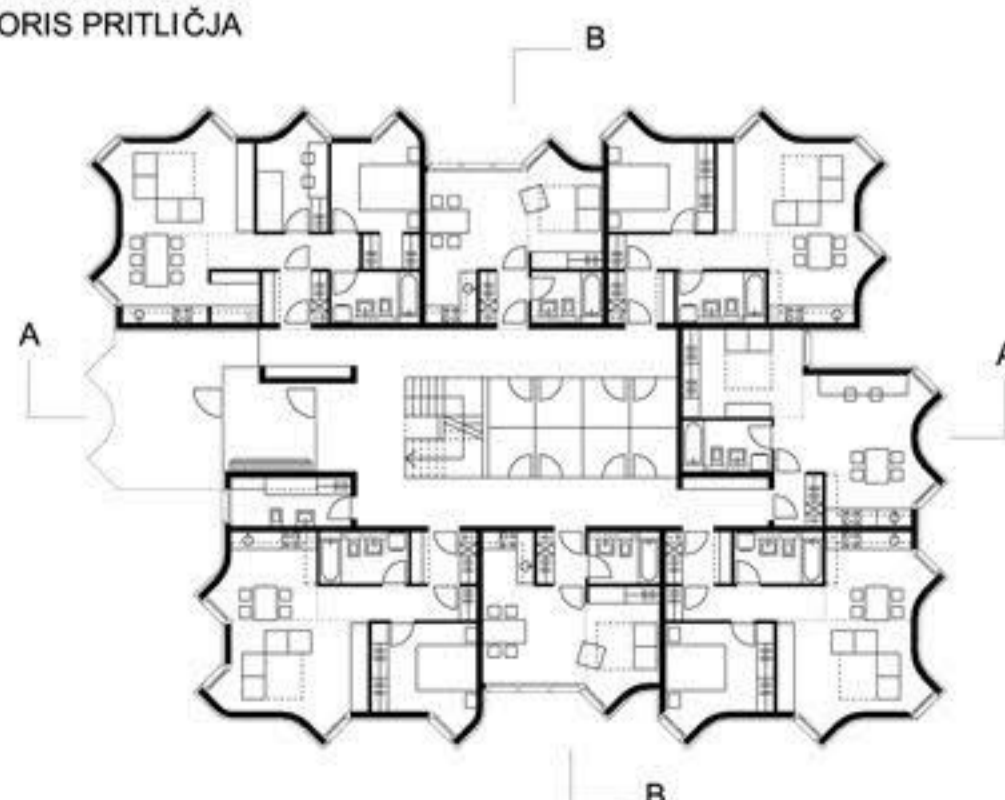
TLORIS PRITLIČJA
