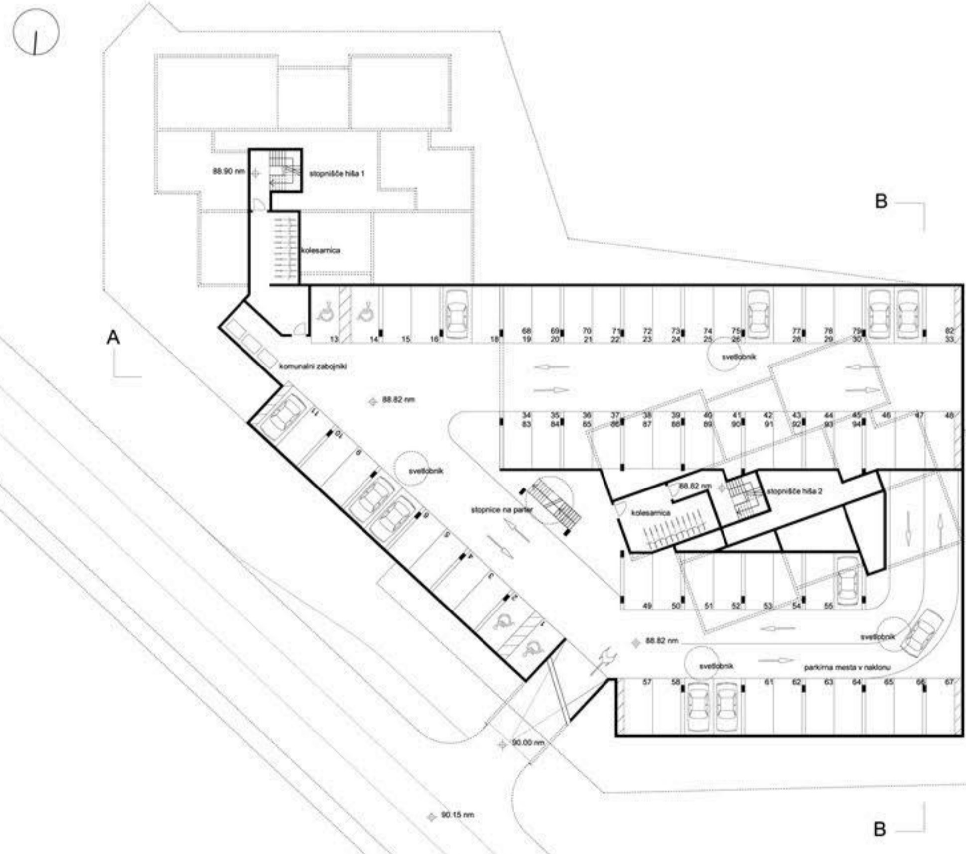
IDEJNA PROMETNA UREDITEV M 1:2000
