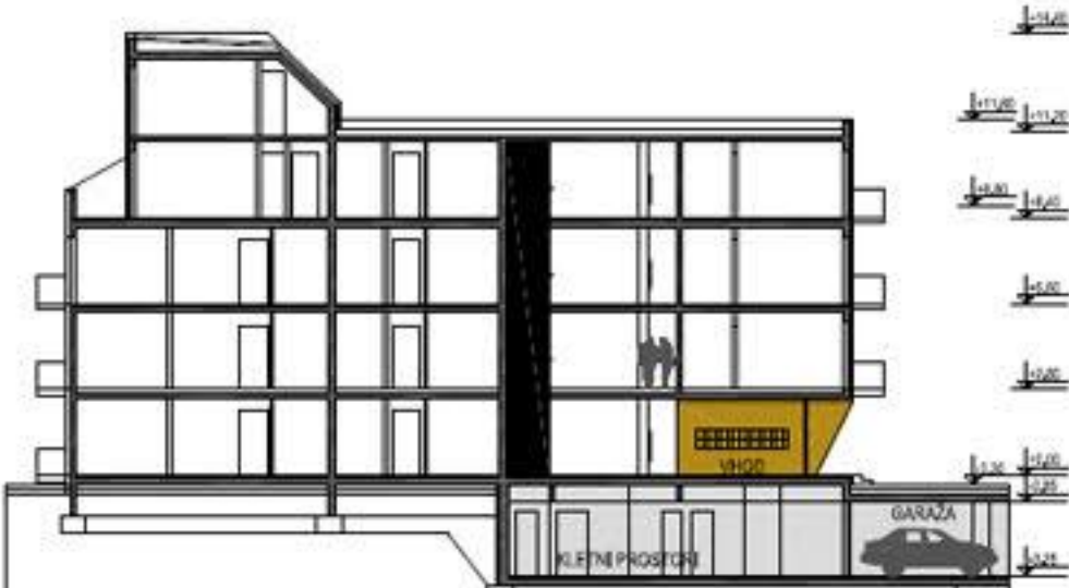
PREČNI PREREZ B-B
