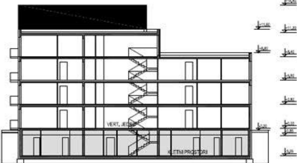
VZDOLŽNI PREREZ AA
