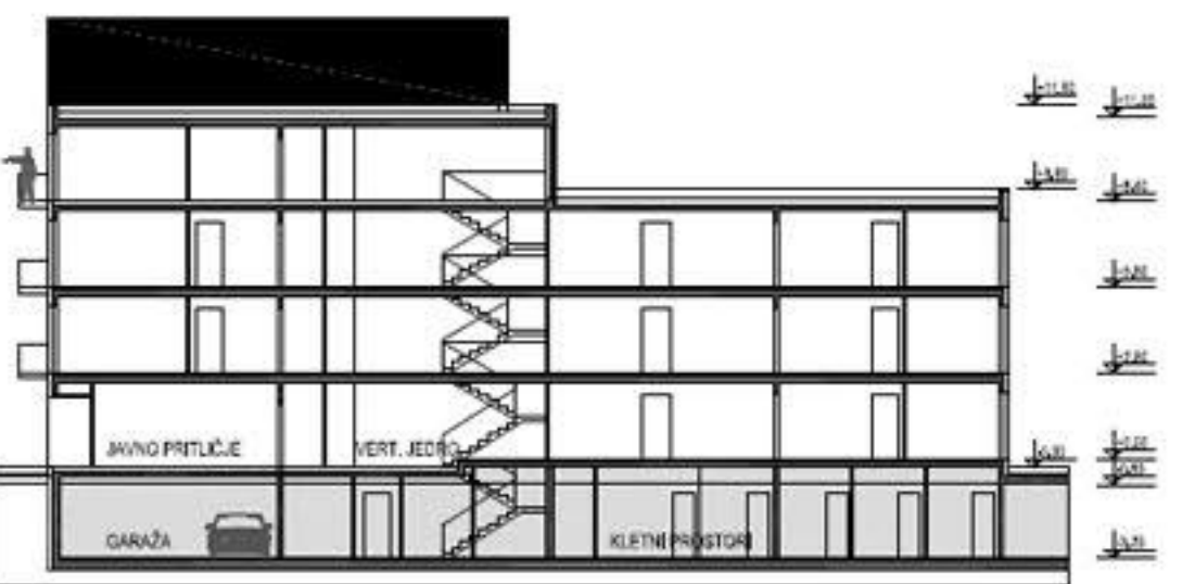
VZDOLŽNI PREREZ AA
