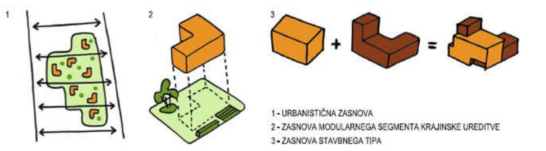
STAVBNI TIP A1-5 - AKSONOMETRIJA
