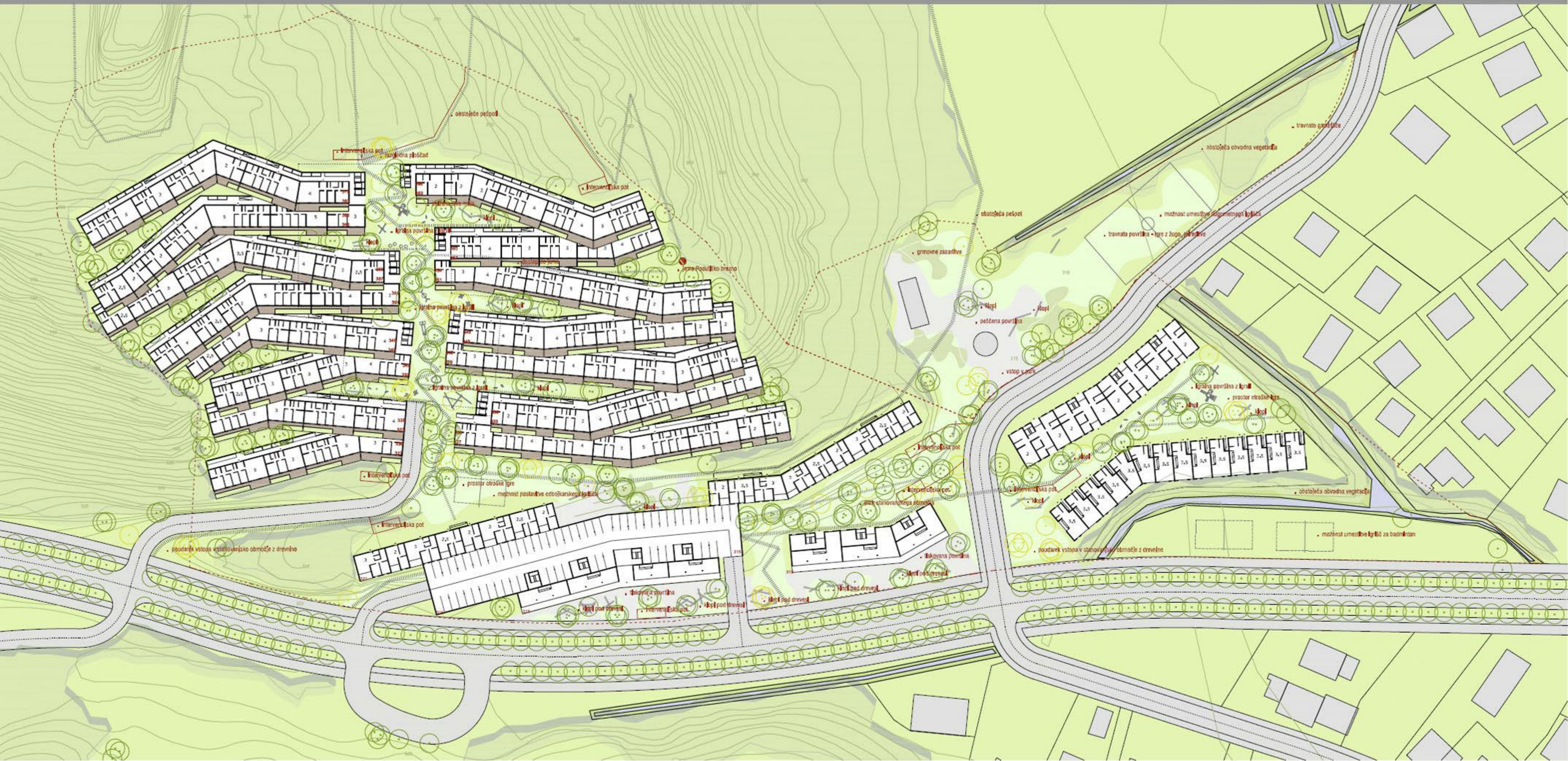
TLORISI GARAŽ m 1:500
