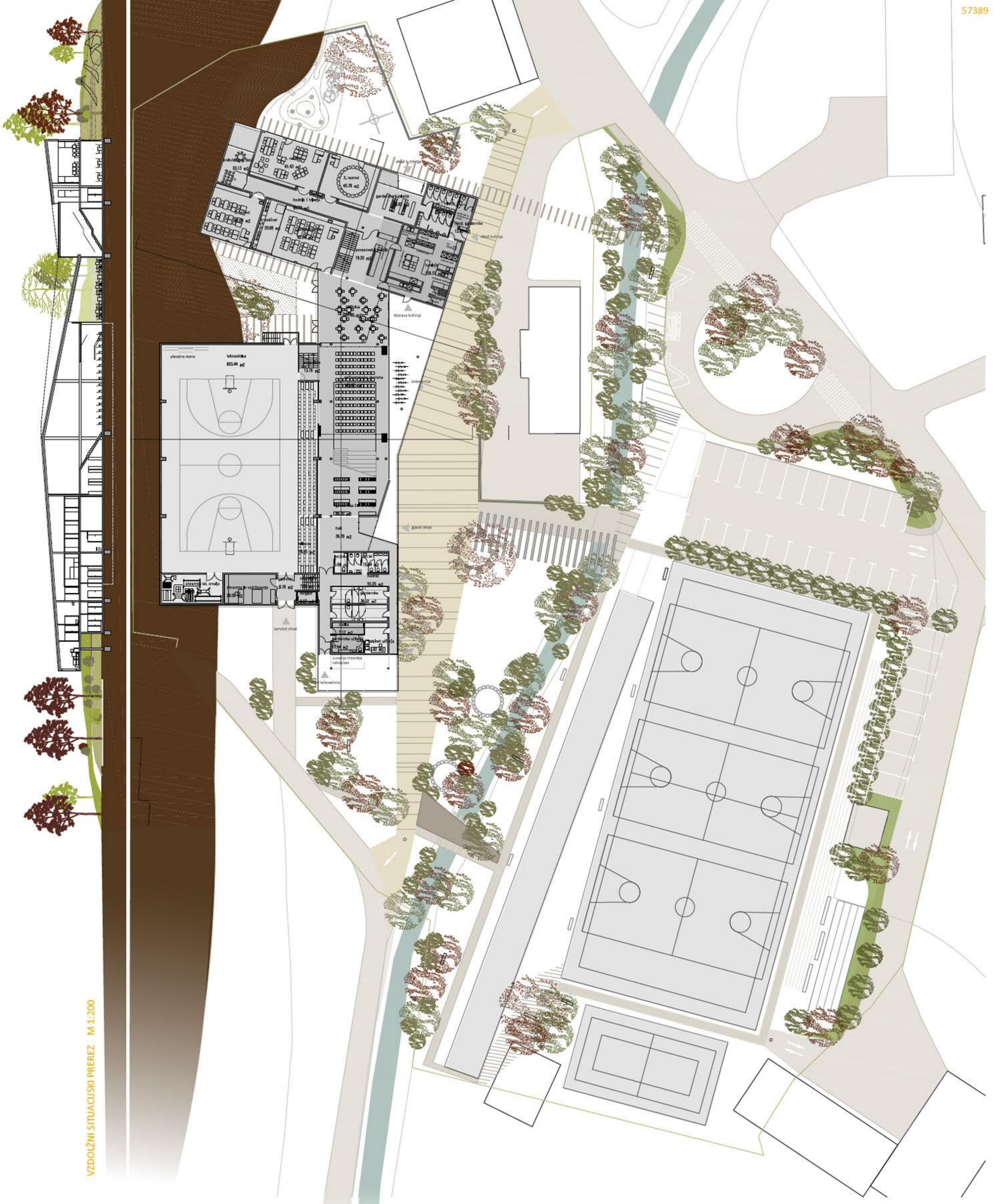
TLORIS PRITLIČJA S SITUACIJO M 1:200
