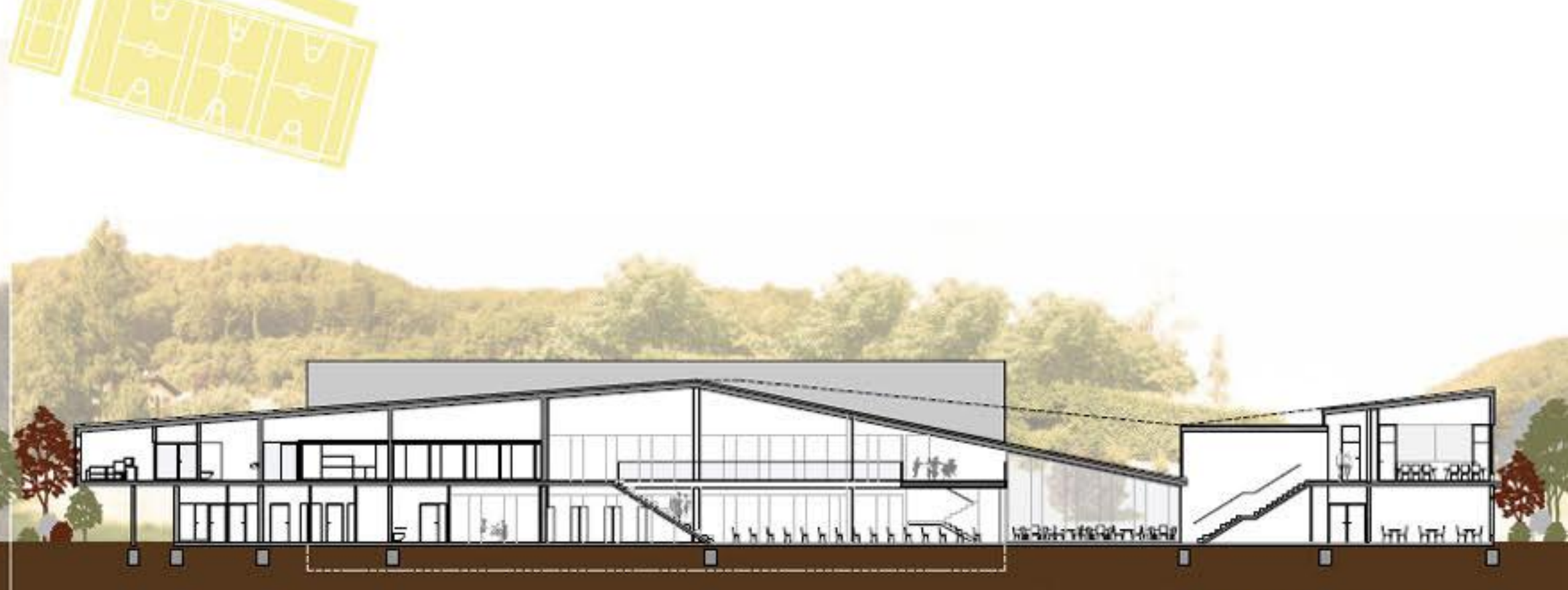
VZDOLŽNI PREREZ M 1:200
