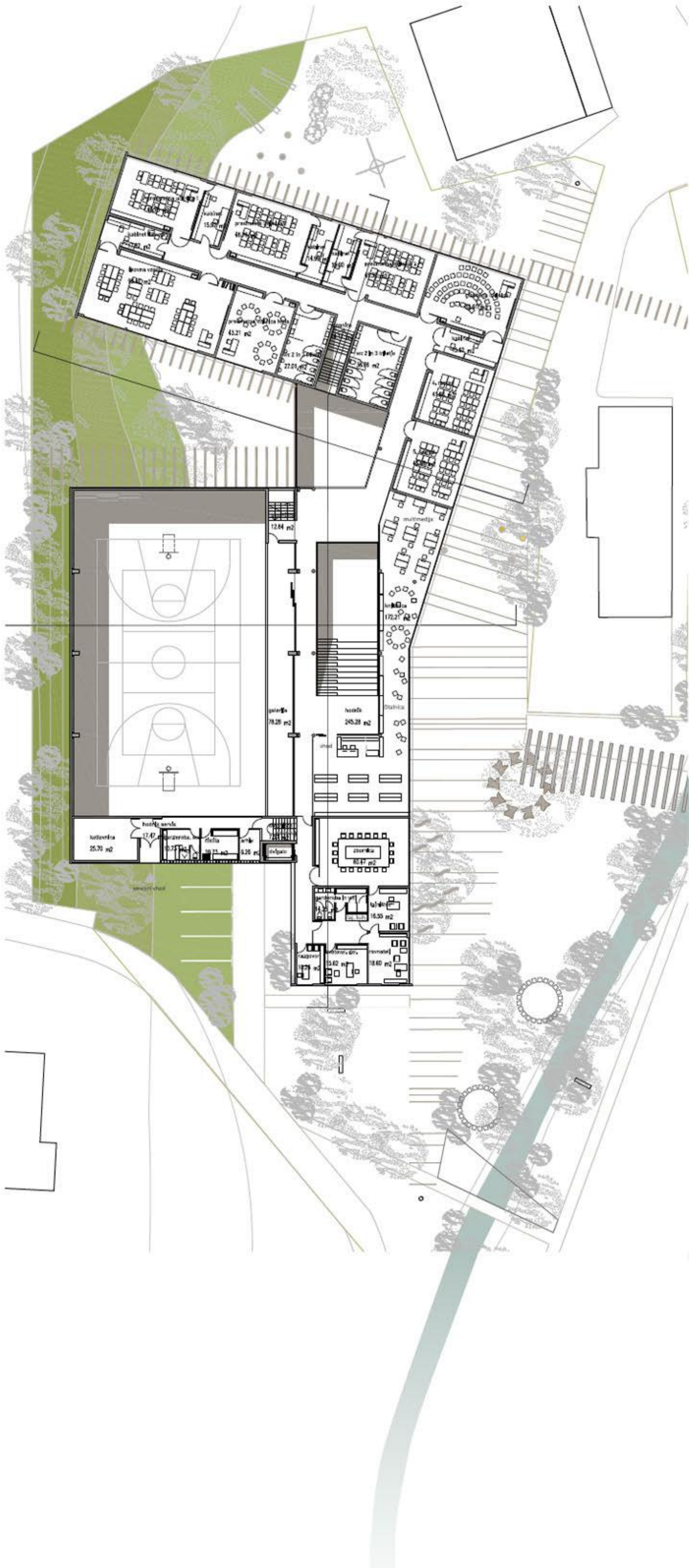
TLORIS NADSTROPJA M 1:200
