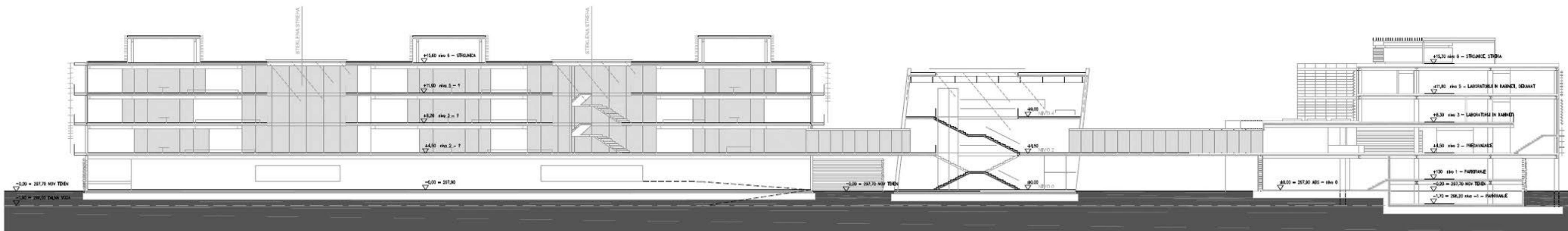
VZDOLŽNI PREREZ SKOZI GLAVNI HALL OBJEKTOV FKKT, X, FRI
