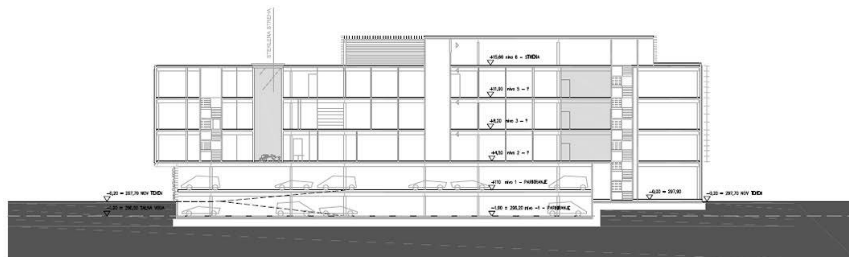
FKKT - PREREZ SKOZI LABORATORIJE
