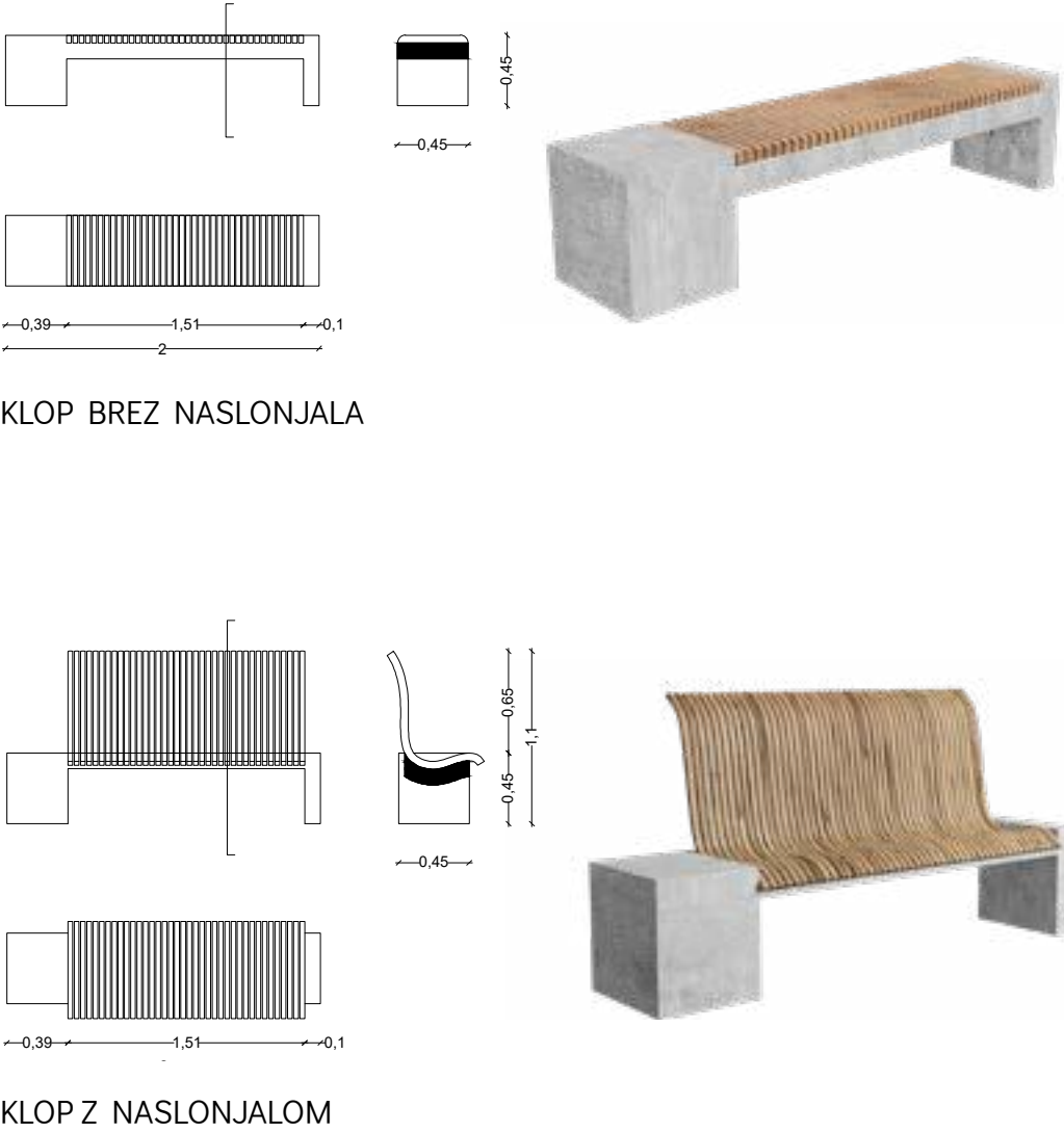
NAČRT URBANE OPREME m 1:50
