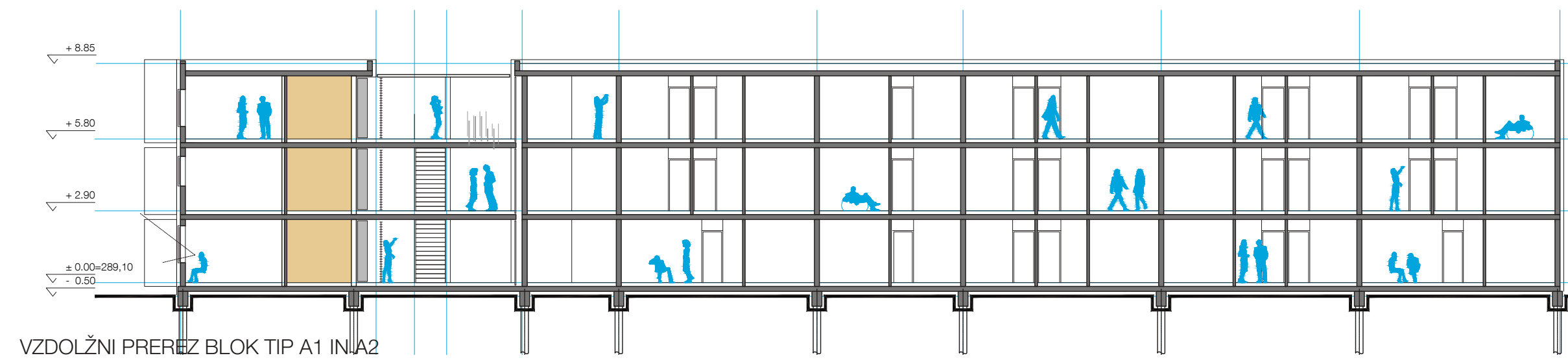
VZDOLŽNI PREREZ BLOK TIP A1 IN A2
