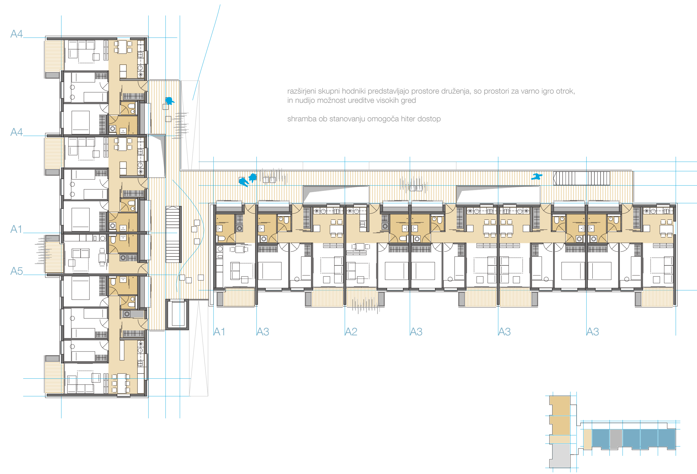
struktura stanovanj po etažah BLOK TIP A1
