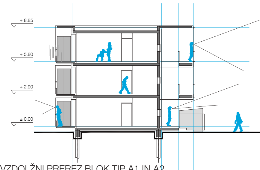
VZDOLŽNI PREREZ BLOK TIP A1 IN A2
