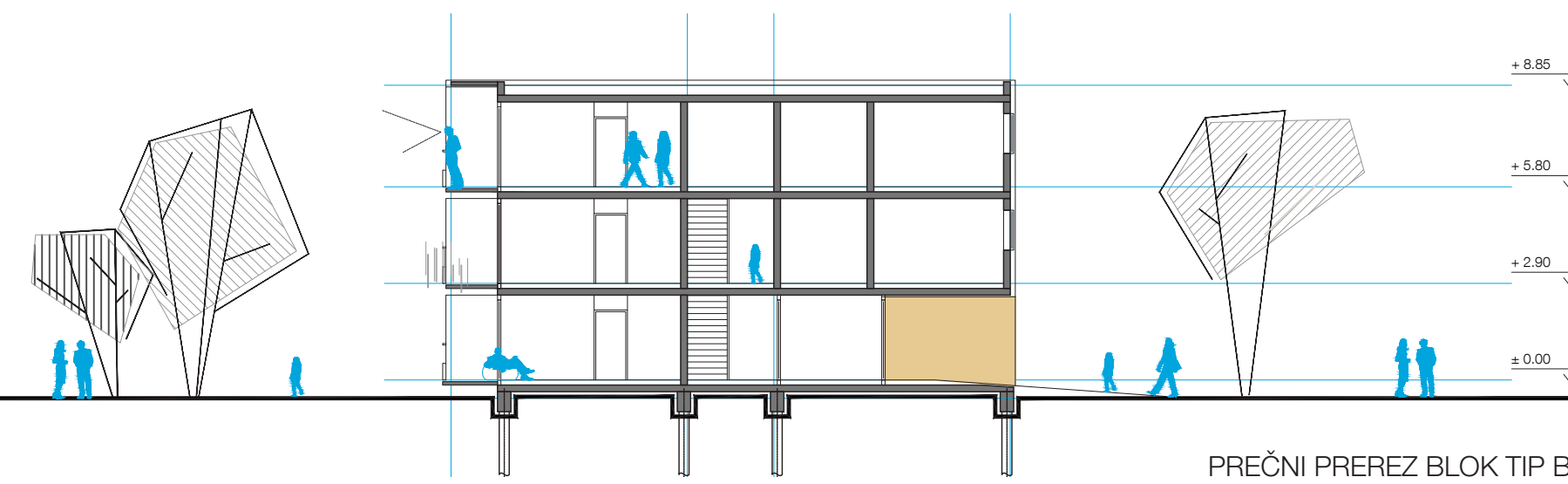
PREČNI PREREZ BLOK TIP B1
