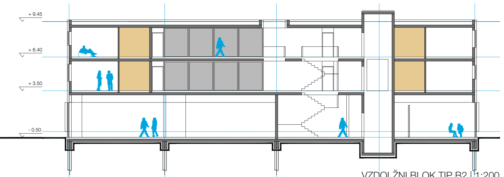
VZDOLŽNI BLOK TIP B2 | 1:200
