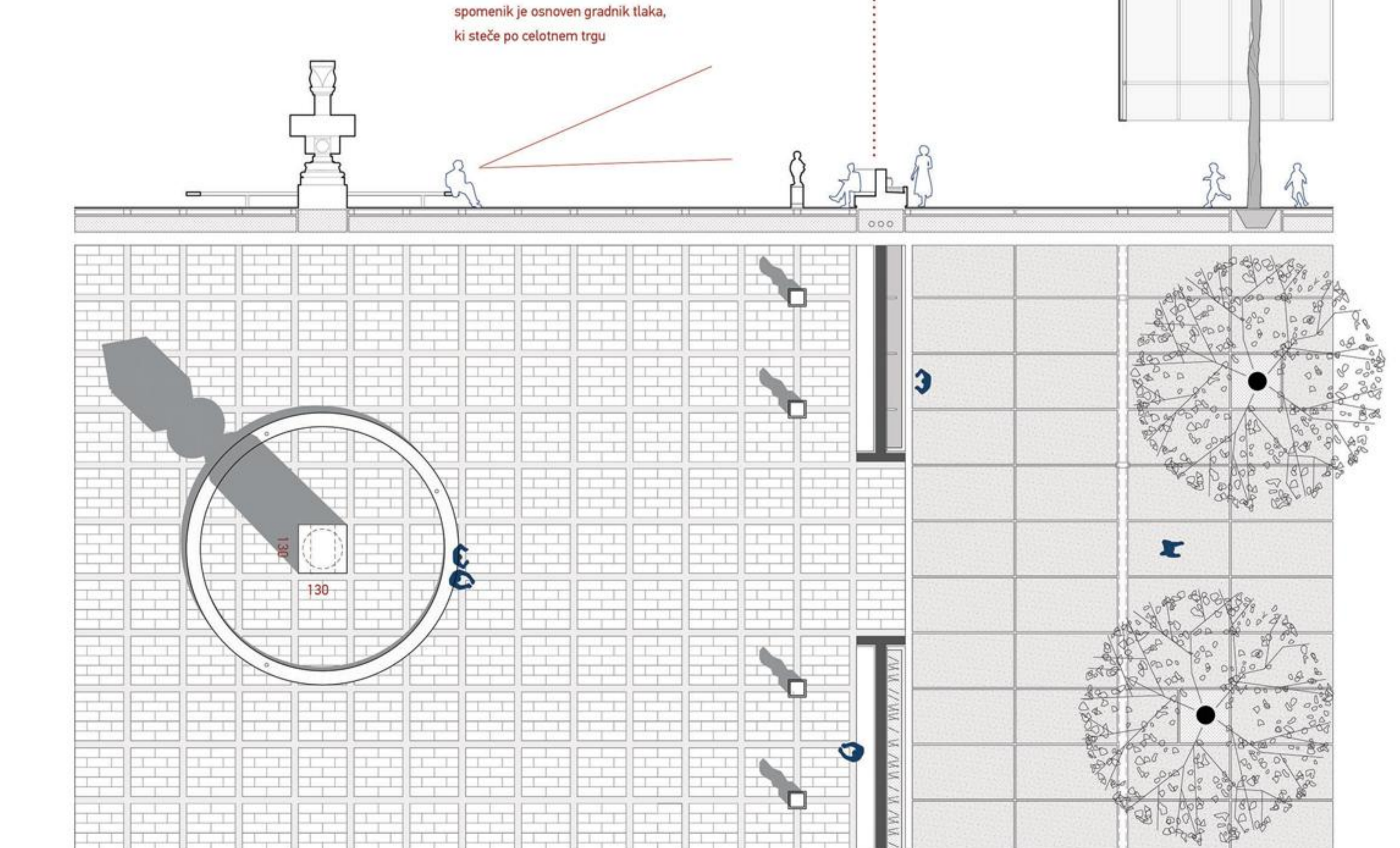
detalji izteka trga s Plečnikovim spomenikom v sekundarni trg s paviljonom 1:100
