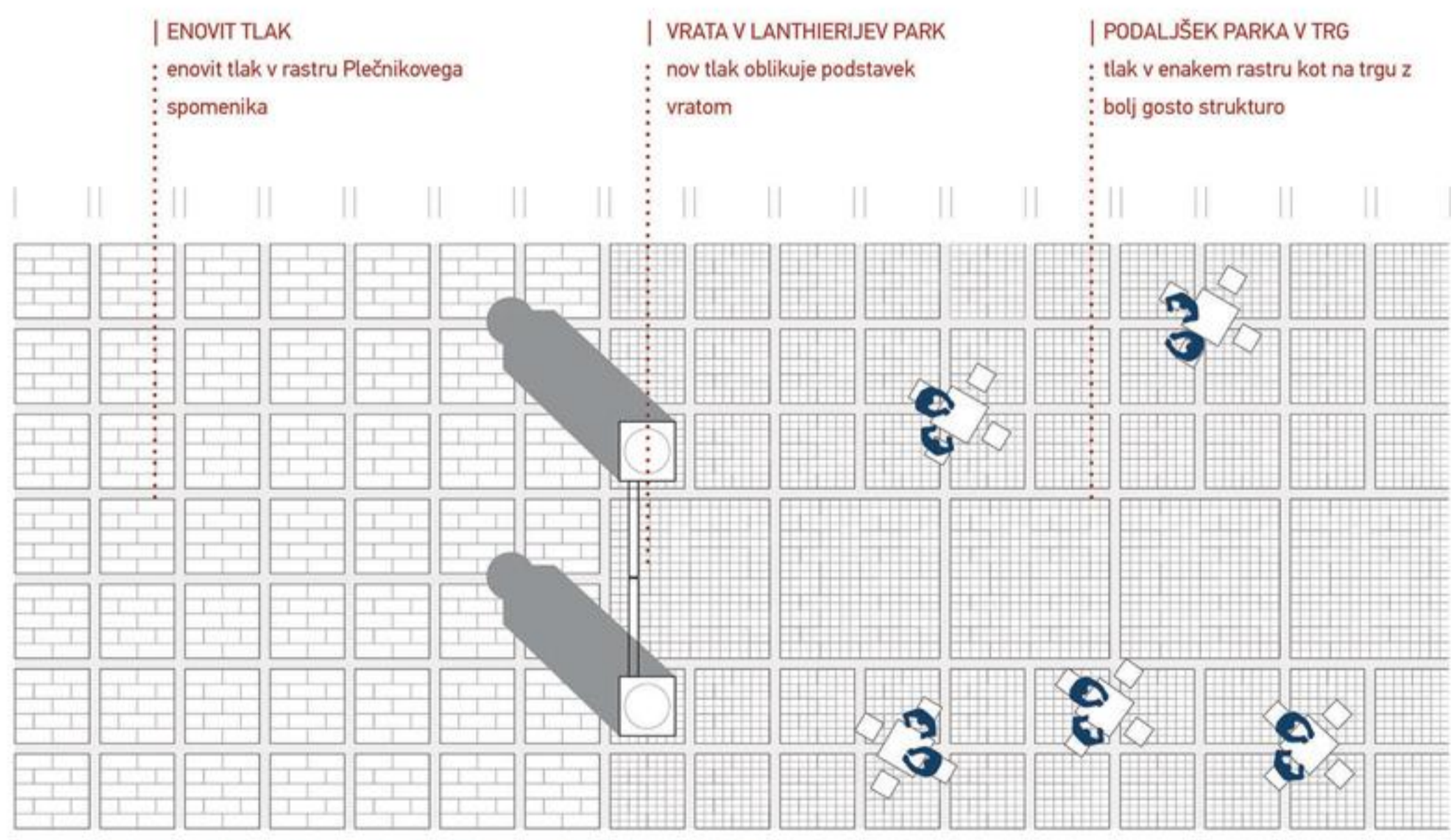
detalji prepleta trga z podaljškom Lanthierjivega parka 1:100
