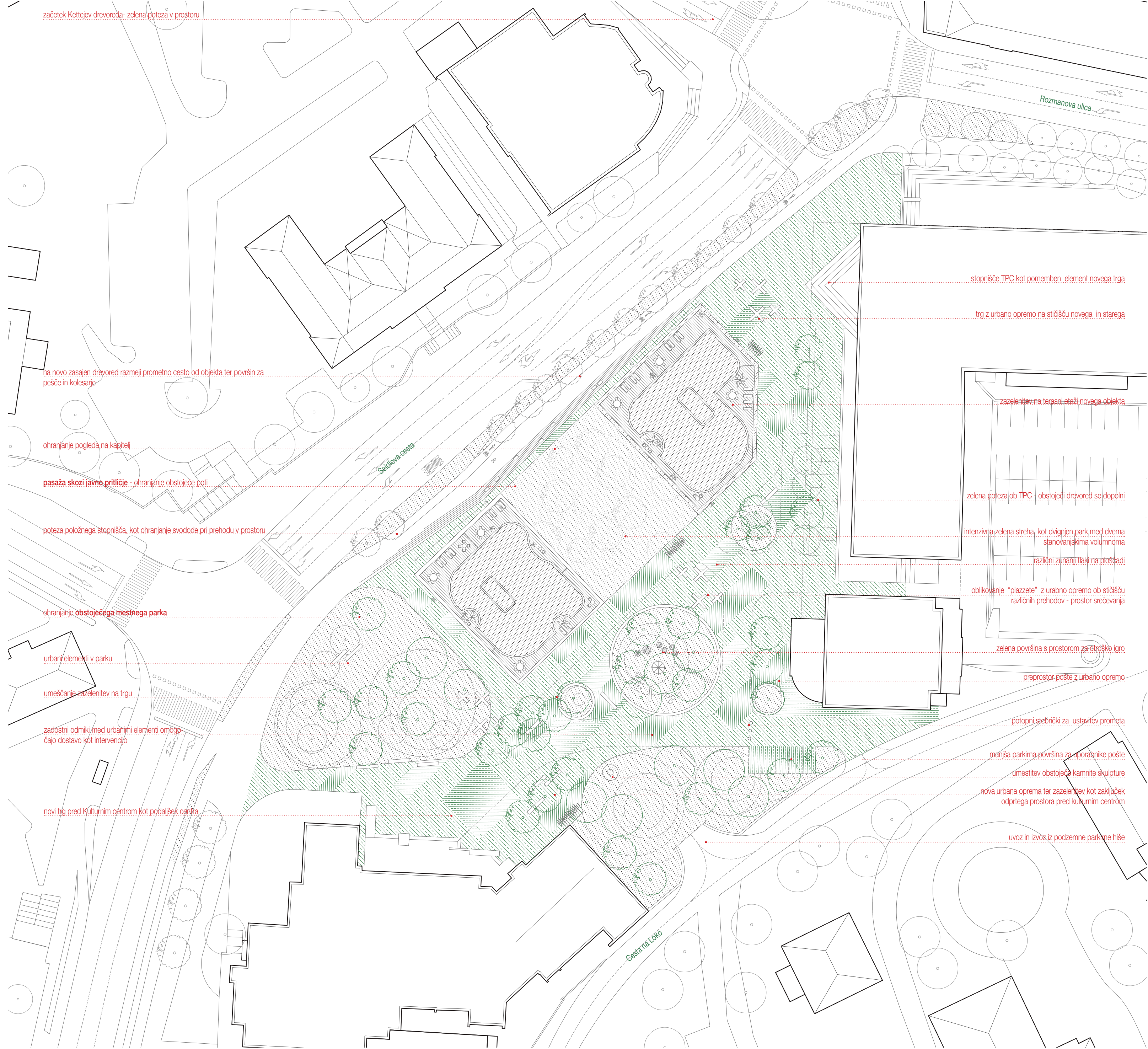
Situacija z ureditvijo ploščadi med objekti 1:500
