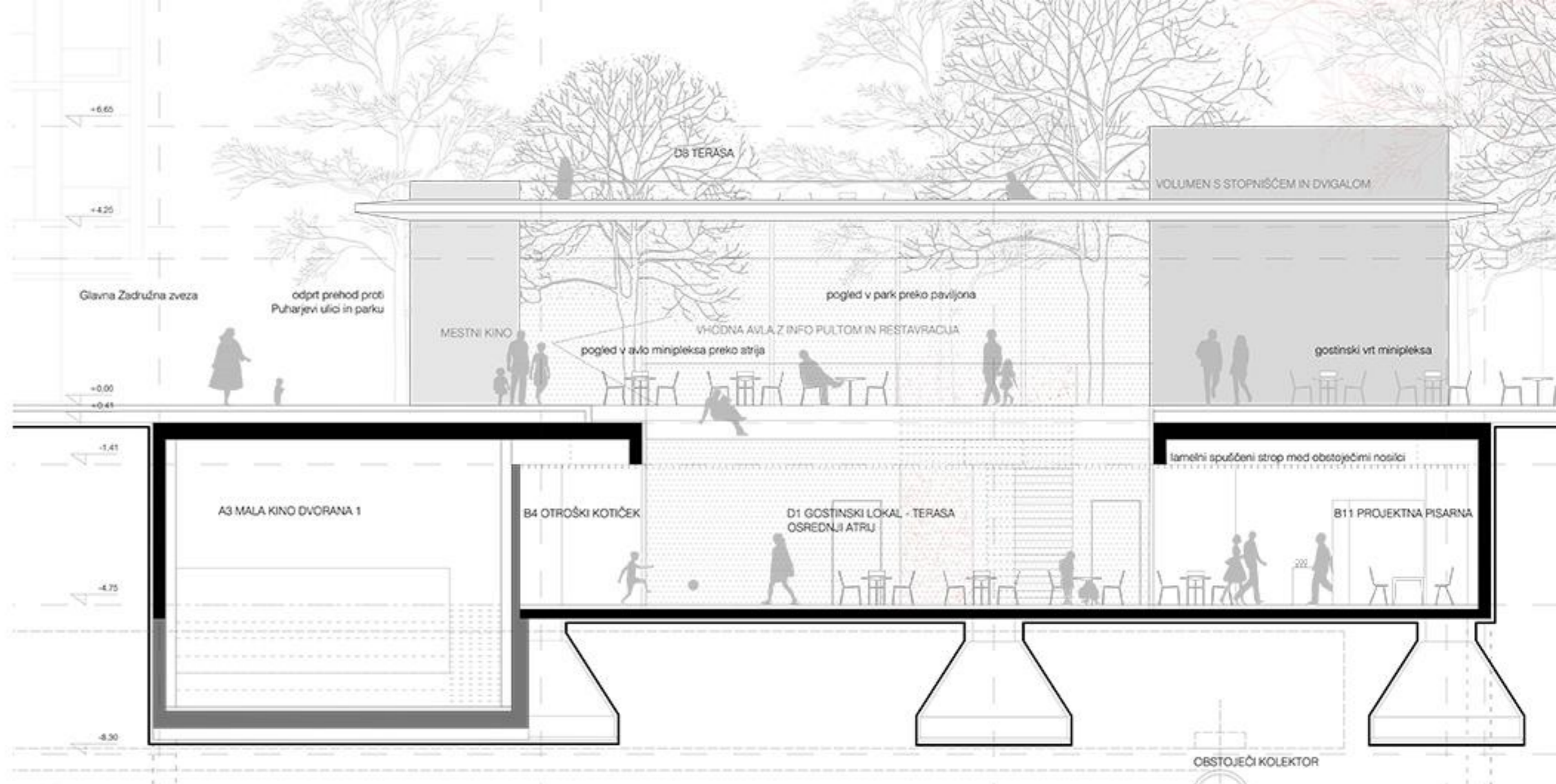
PREČNI PREREZ IN VZHODNA FASADA 1:100
