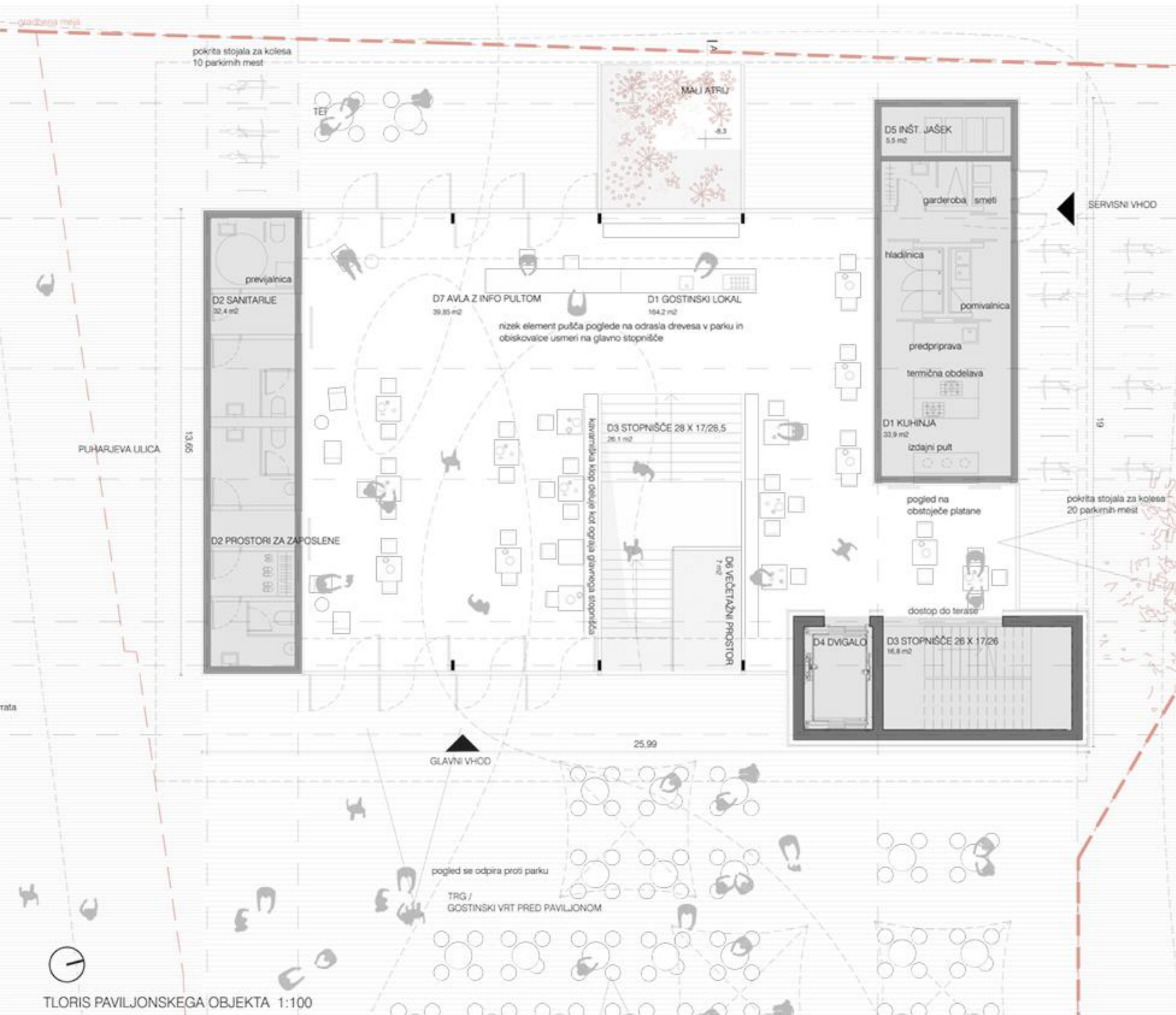
TLORIS PAVILJONSKEGA OBJEKTA 1:100
