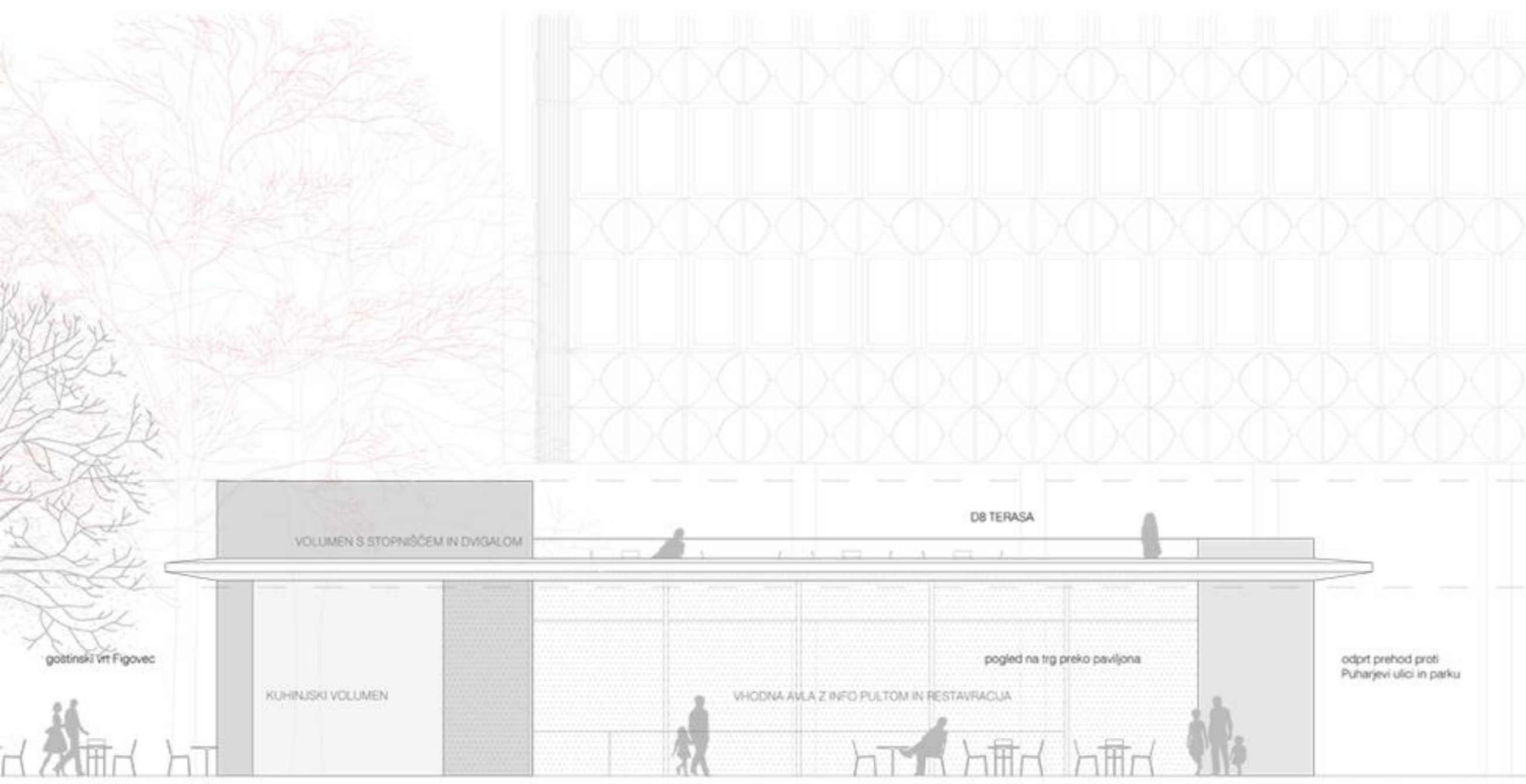
ZAHODNA FASADA NADZEMNEGA DELA OBJEKTA
