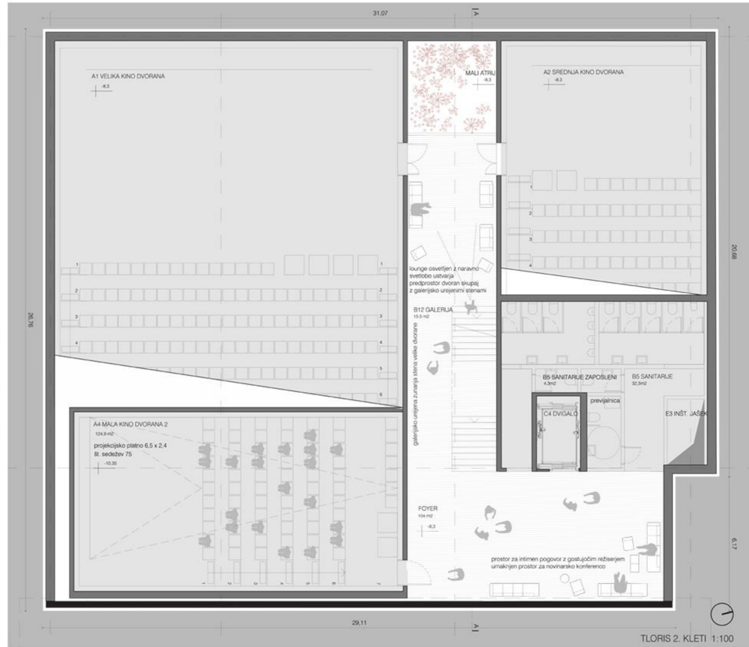
TLORIS 2. KLETI 1:100
