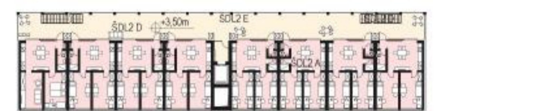
Tloris tipične etaže ŠDL 2, M 1:500
