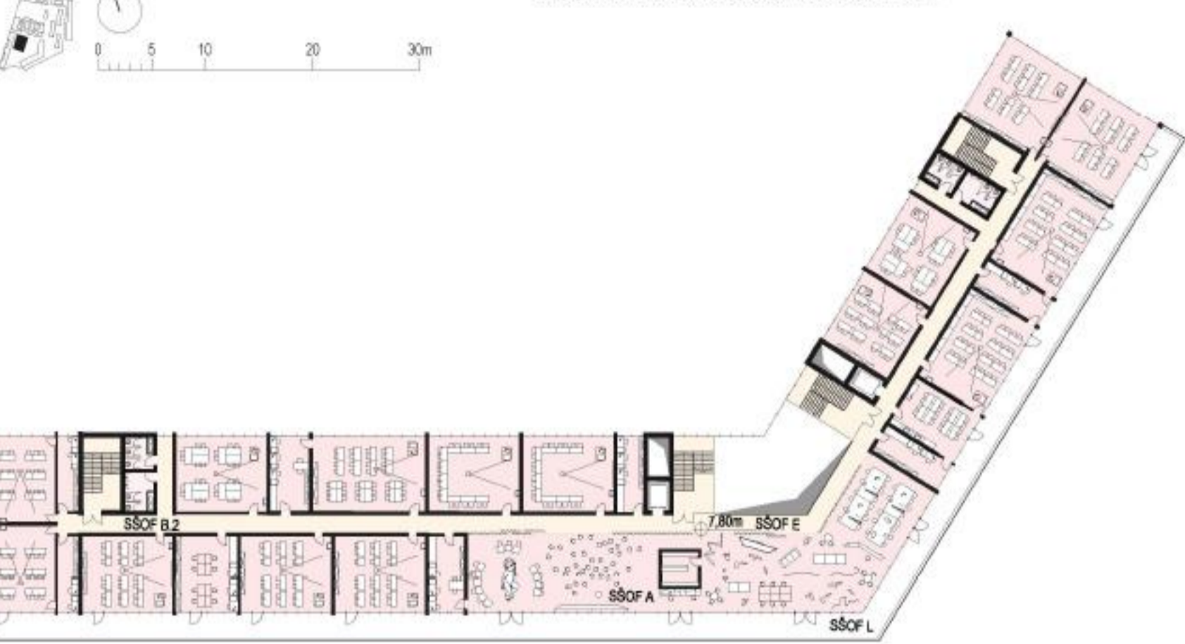
Tloris 2. nadstropja SŠOF, M 1:500
