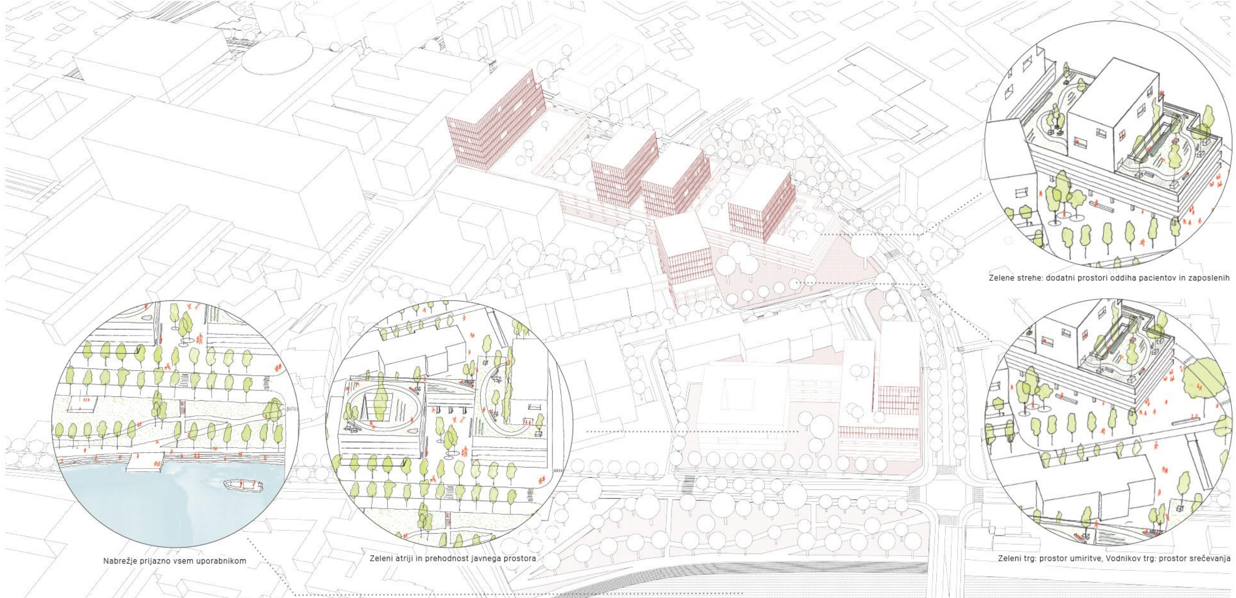
AKSONOMETRIČNI PRIKAZ
