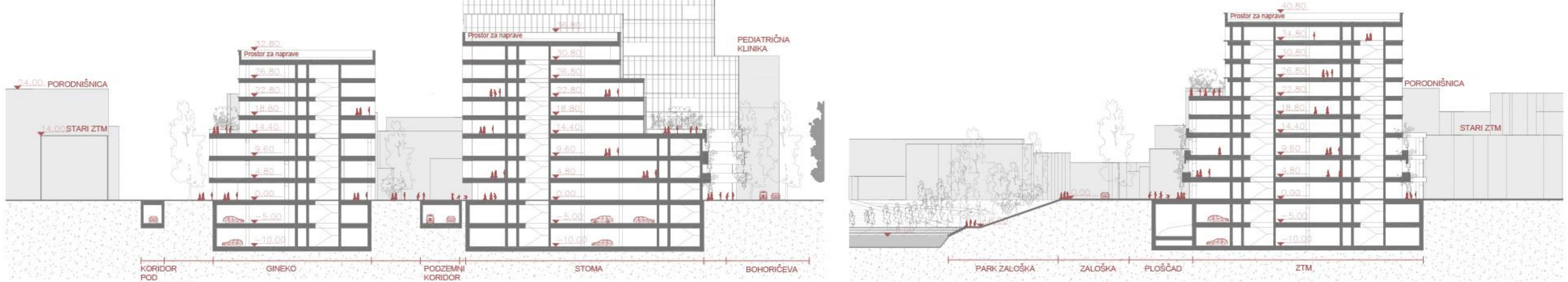
PREČNI PREREZ B-B M: 1:500
