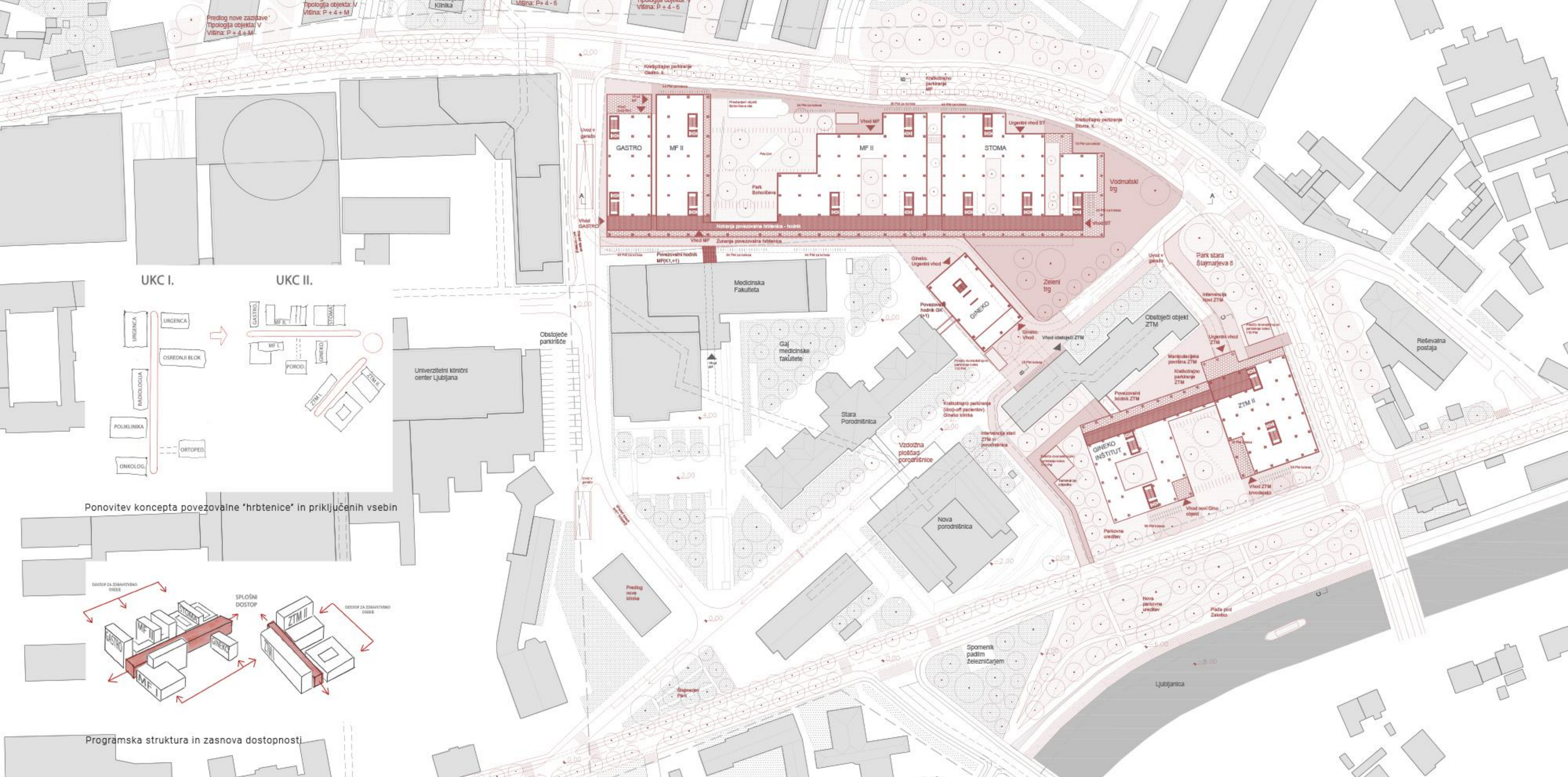
UREDITVENA SITUACIJA ŠIRŠEGA NATEČAJNEGA OBMOČJA M: 1:1000
